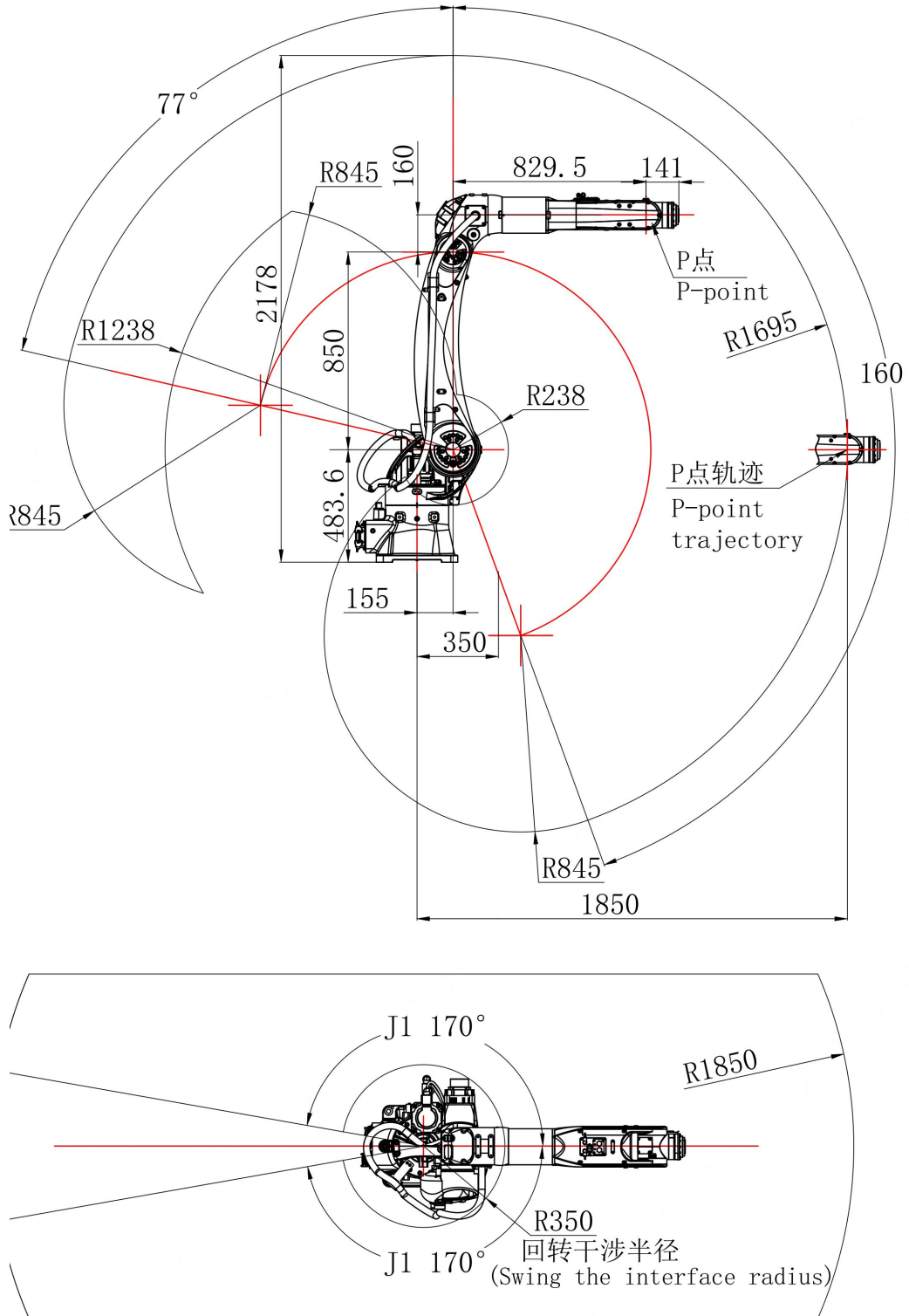
图 2-8 机器人工作空间图
