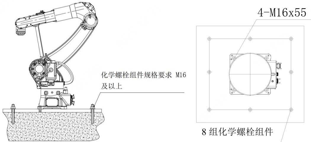
图 3-11 机器人安装举例
