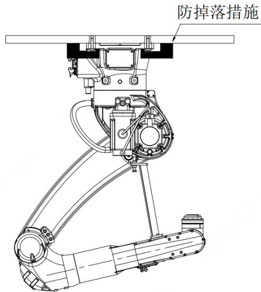
图 3-12 倒挂安装
