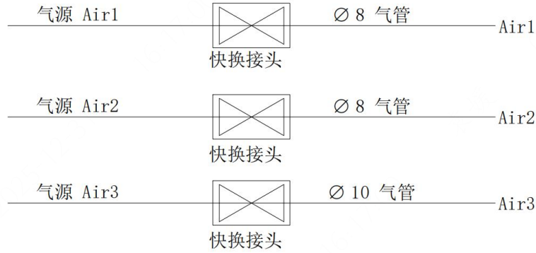
图 3-21 标准型气路原理图 (标准)
