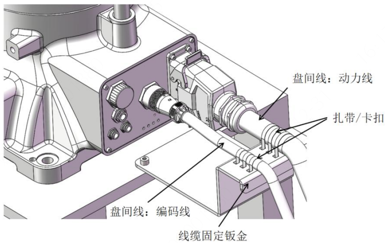
图 3-6 机器人盘间线固定示意图
