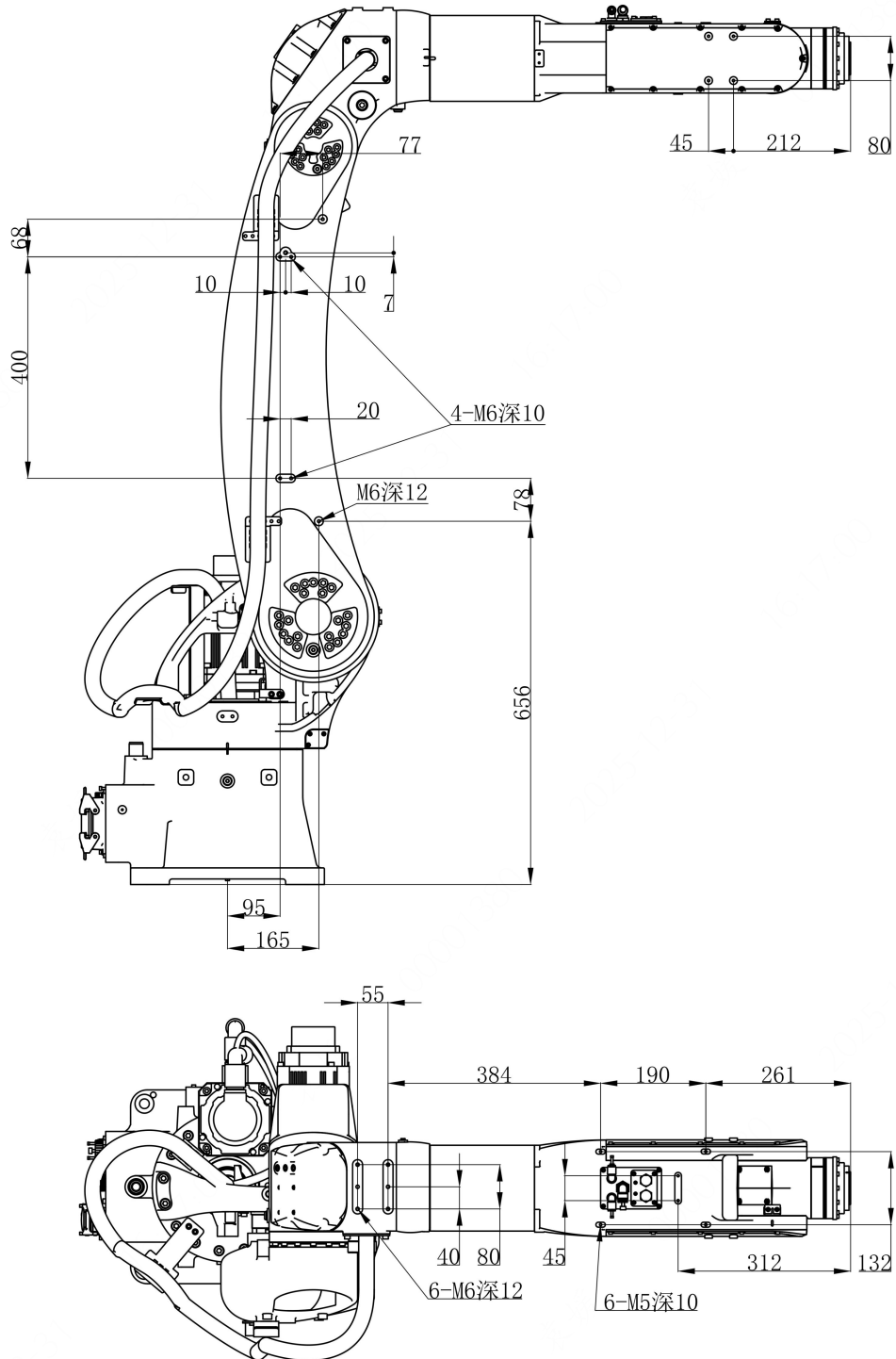
图 3-15 外围安装尺寸图
