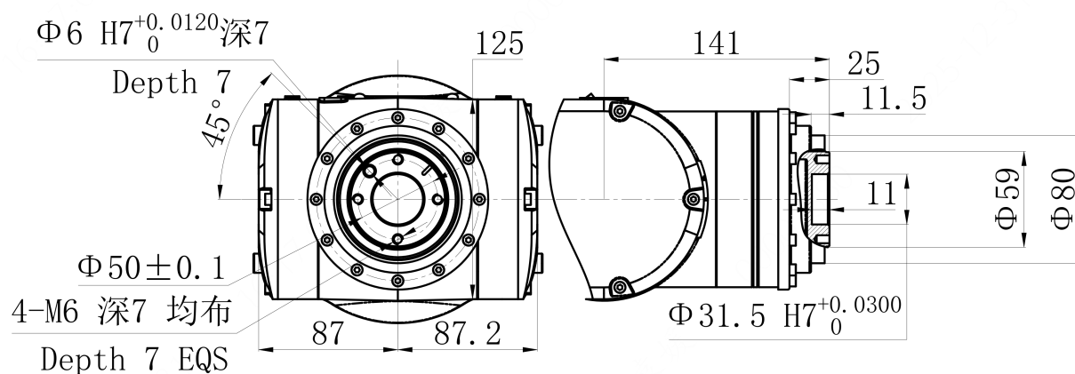
图 3-14 末端负载安装法兰尺寸
