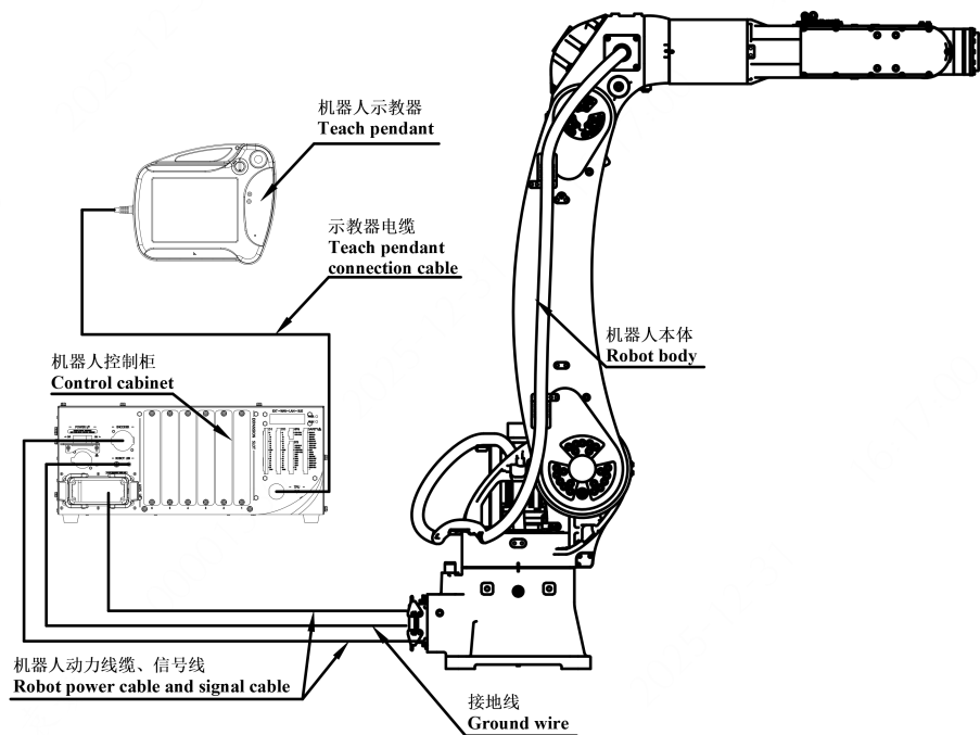
图 2-1 工业机器人系统构成
