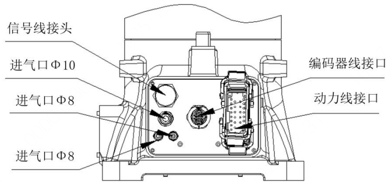
图 3-22 底座部分气路及信号线接口
