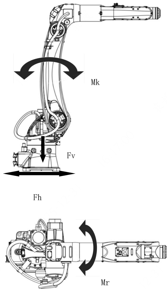
图 3-13 机器人受力图
