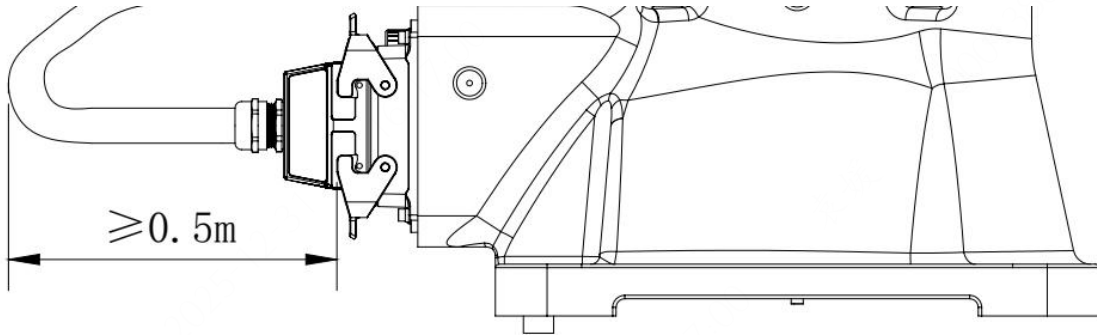
图 3-8 底座线缆后侧出线最小弯折尺寸
