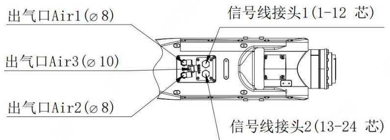
图 3-23 小臂部分气路及信号线接口
