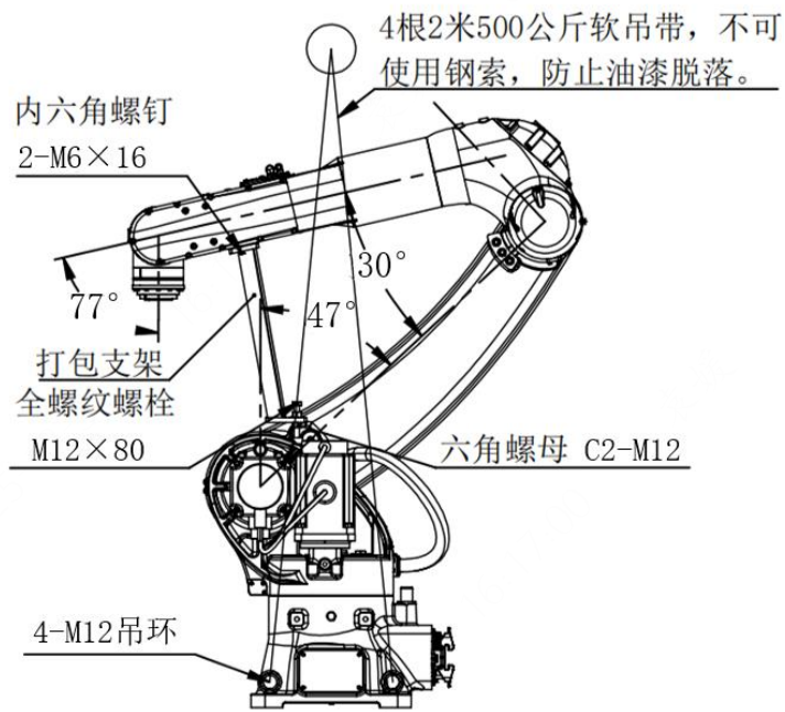
图 3-3 吊装搬运示意图
