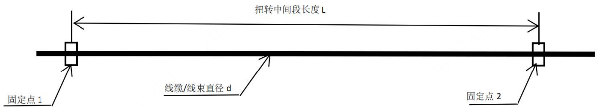
图 3-9 线缆/线束扭转距离
