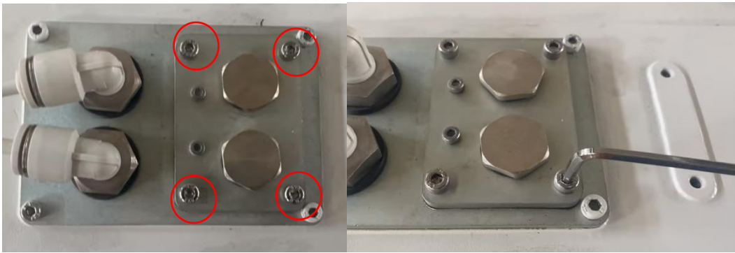
图 3-17 I/O 顶盖螺钉拆卸示意图
