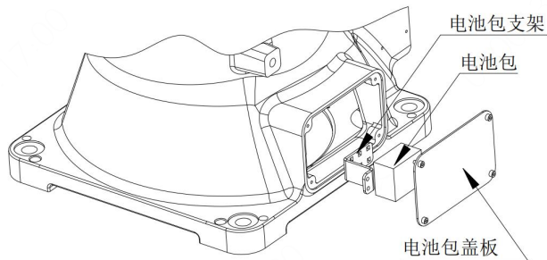
图 4-5 机器人电池组位置图
