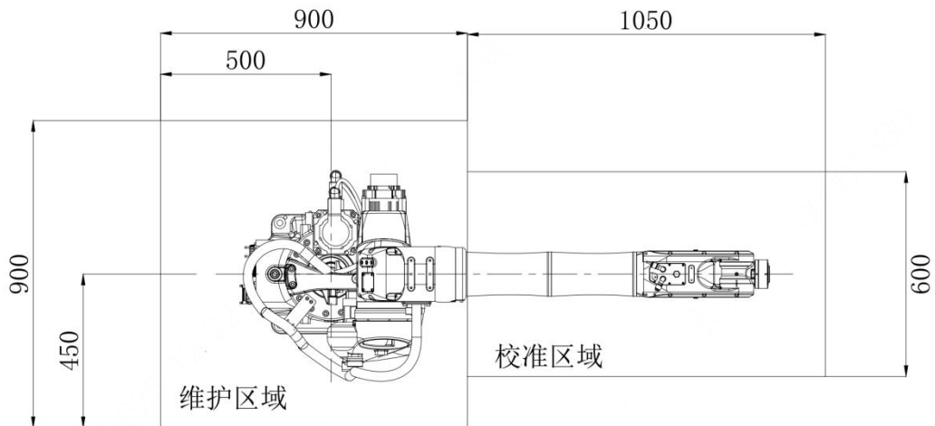
图 4-4 维护及使用区域
