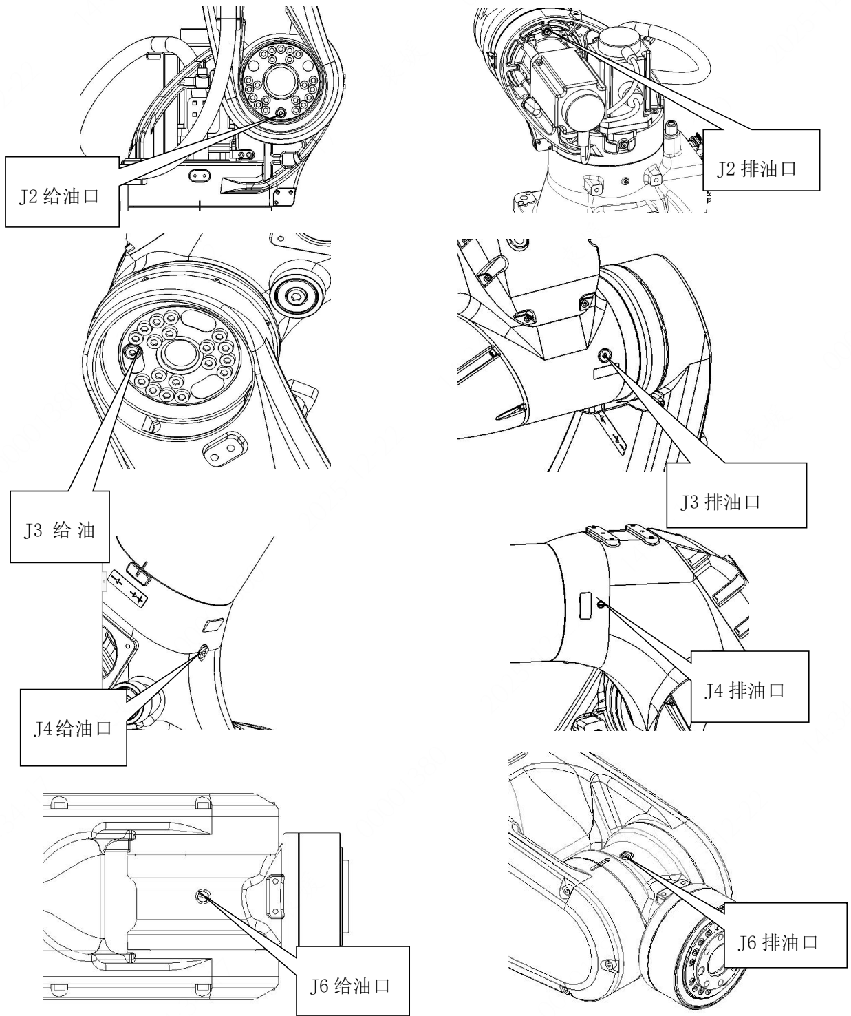
图 4-1 机器人注油口和排气口分布图
