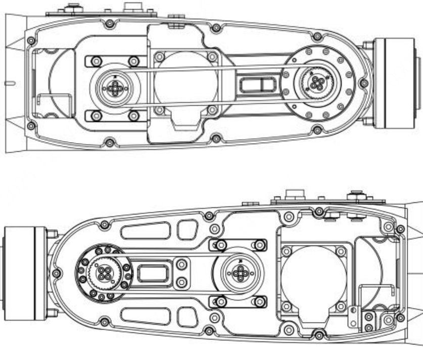
图 4-2 ER12-2100 机器人 J5、J6 轴同步带结构图
