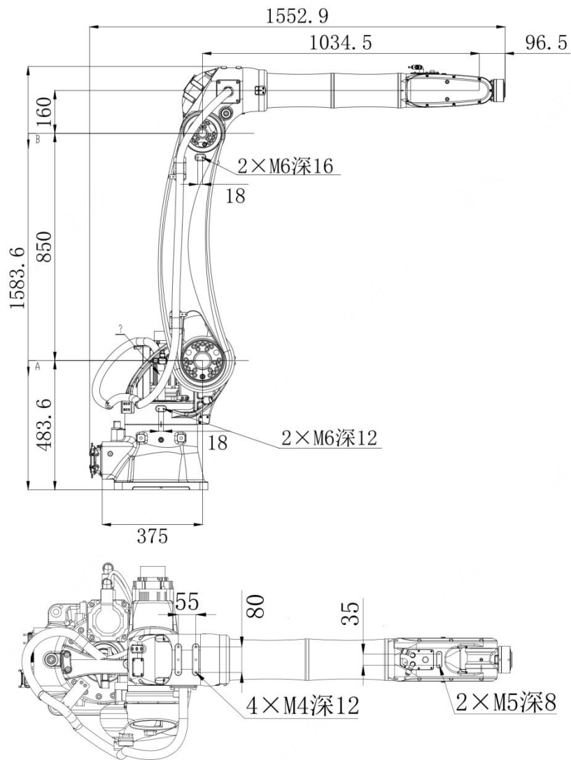
图 3-12 外围安装尺寸图
