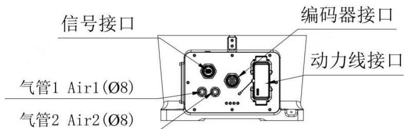
图 3-16 底座部分气路及信号线接口
