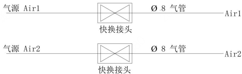
图 3-15 标准型气路原理图（标准）
