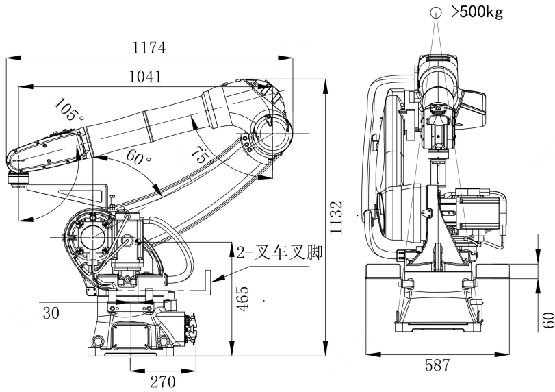
重心位置 3-3 吊装搬运示意图
