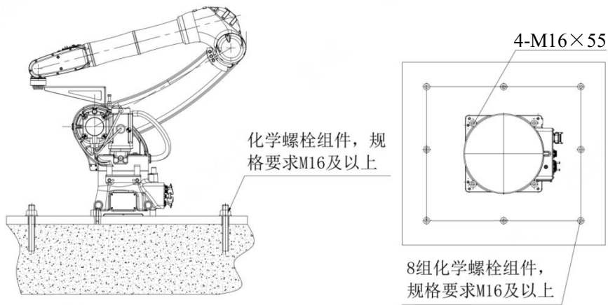
图 3-9 机器人安装举例
