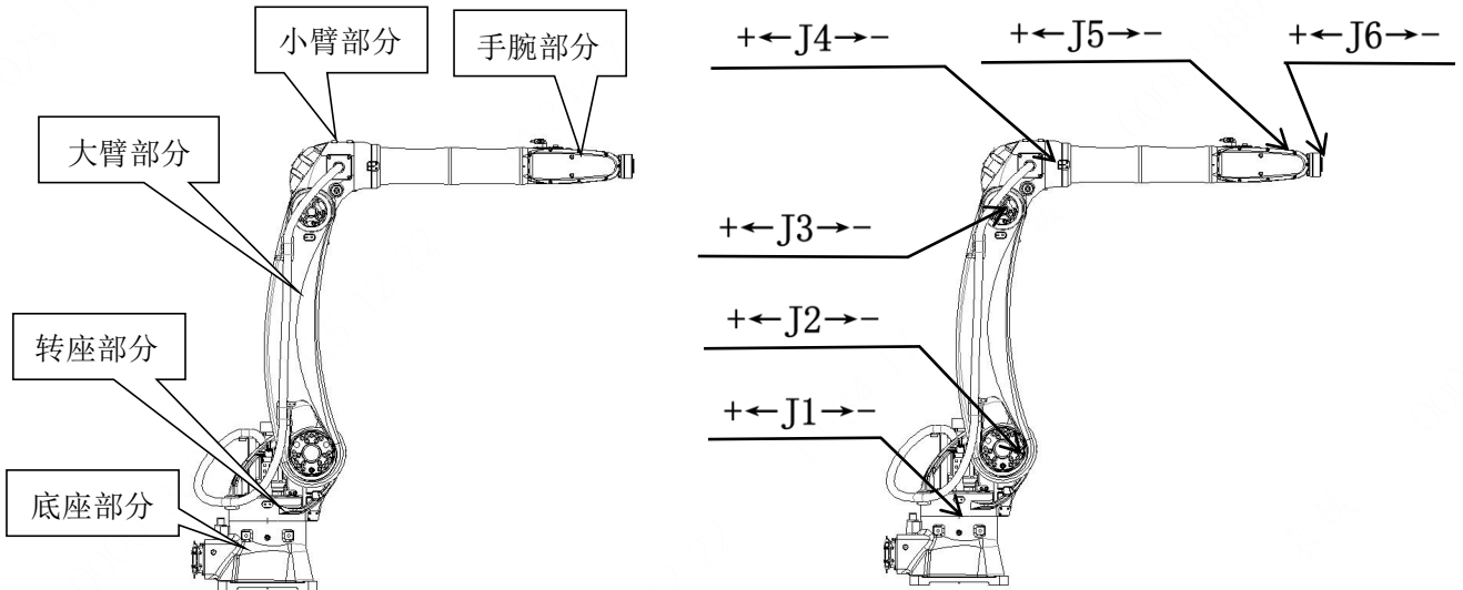
图 2-3 ER12-2100 机械本体组成部分
