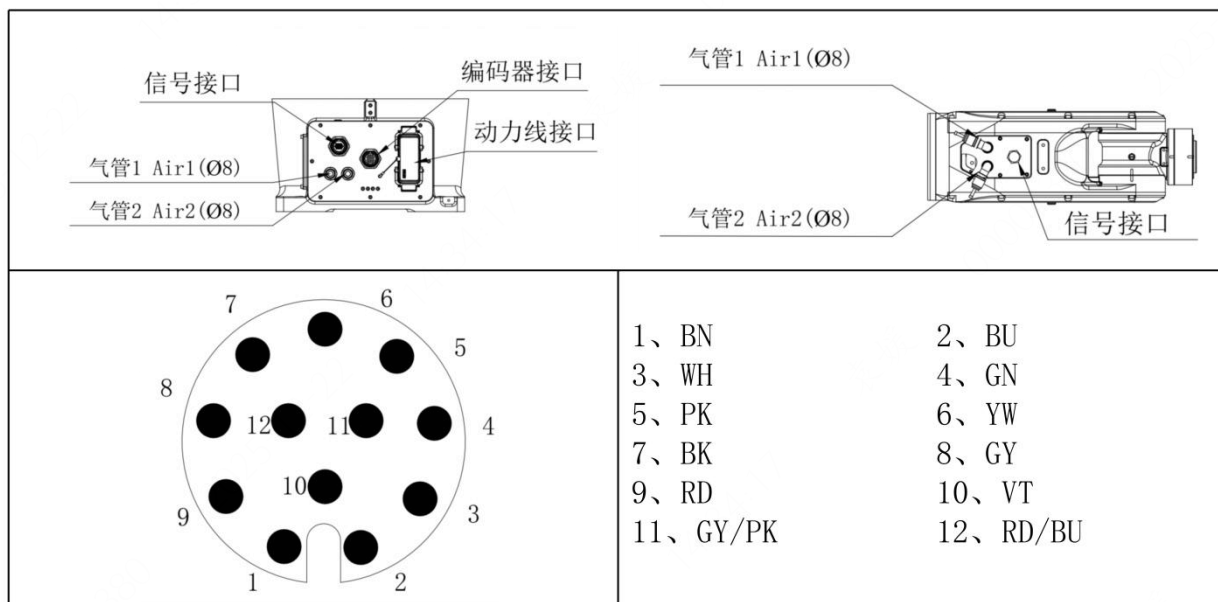
图 3-14 标准型气路信号线位置图
