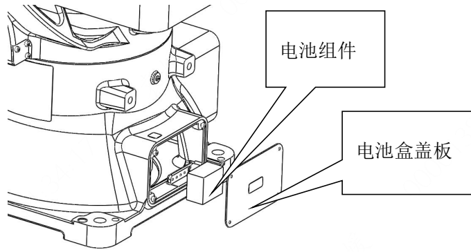
图 4-6 机器人电池组位置图
