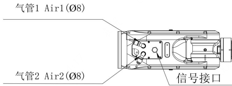
图 3-17 小臂部分气路及信号线接口
