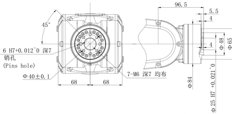
图 3-11 末端负载安装法兰尺寸
