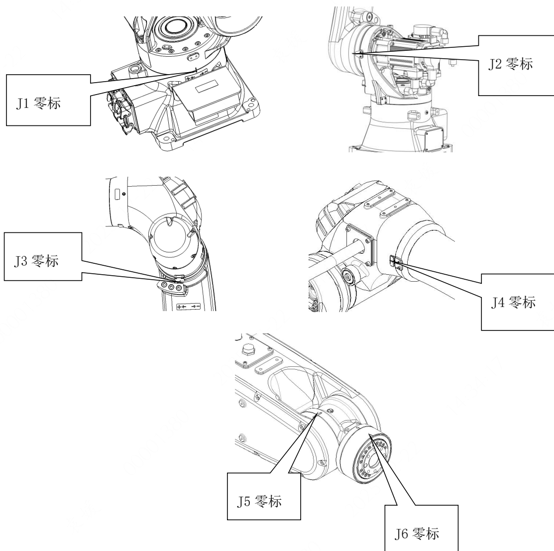
图 4-5 机器人零点位置图
