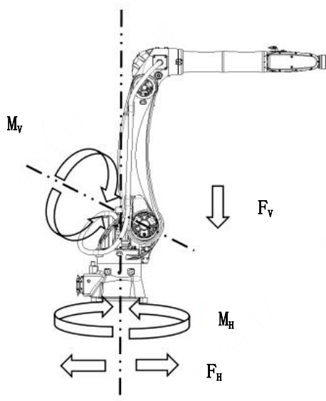
图 3-10 机器人受力图
