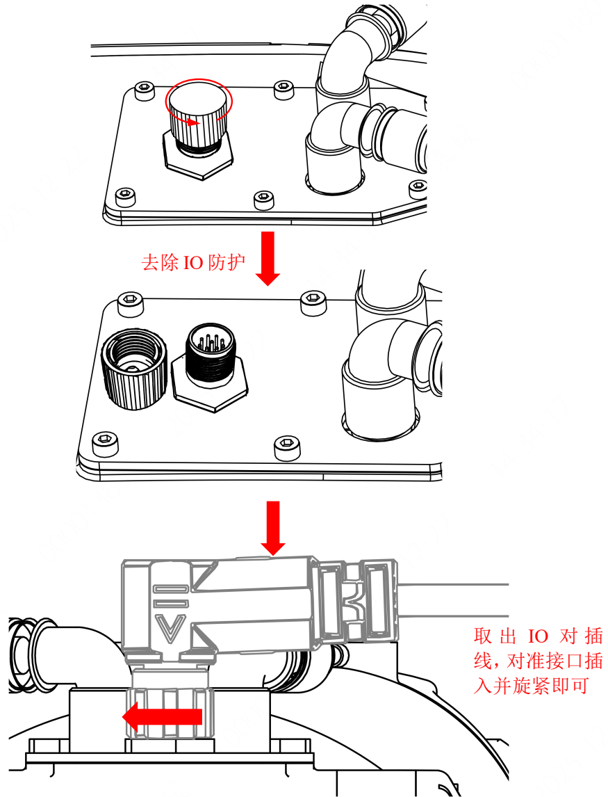
图 3-13 I/O 线对接流程
