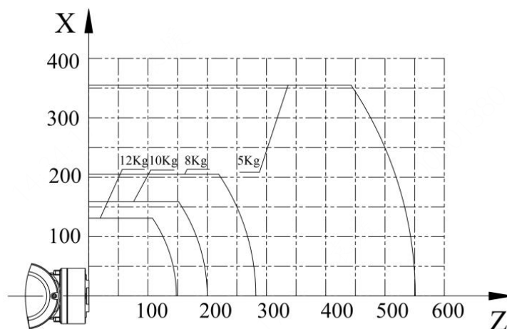
图 2-6 ER12-2100 手腕轴转矩图
