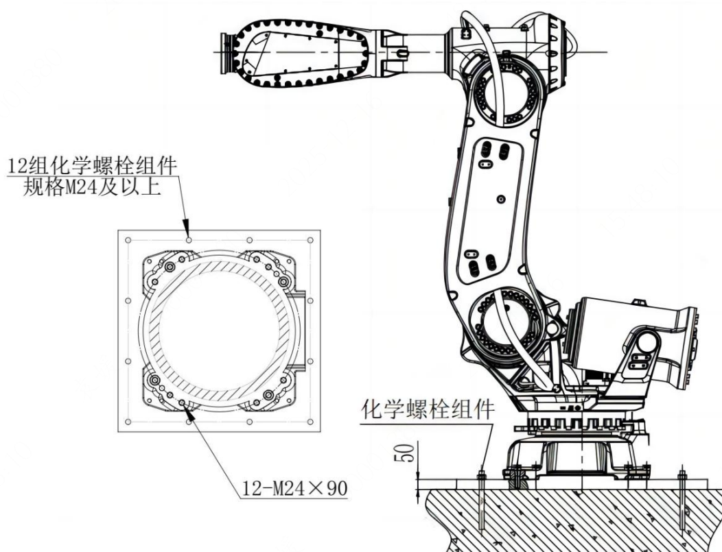
图 3-9 机器人安装举例
