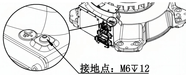
(b) 接地点示意图
