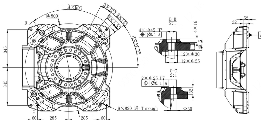
图 3-5 机器人底座尺寸
