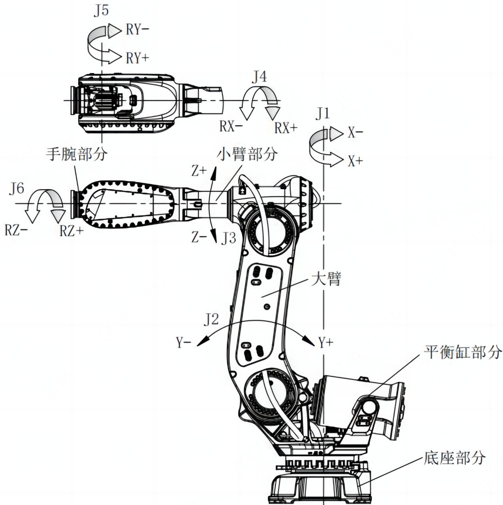
图 2-3 ER360 系列机械本体组成部分
