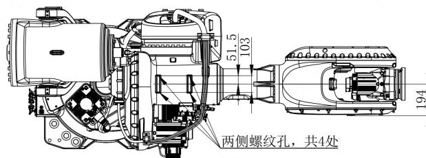
(a) ER360-2800 & ER280-3200
