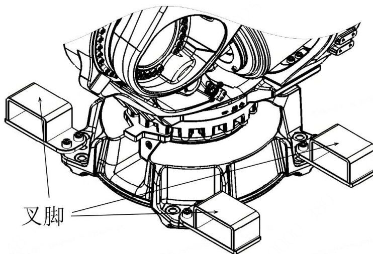
图 3-2 叉脚安装示意图
