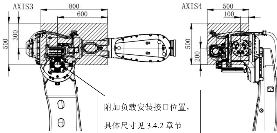
图 2-8 ER360 系列上臂附加负载质心范围图
