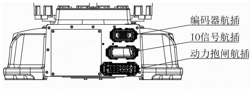
图 3-15 底座部分信号线接口
