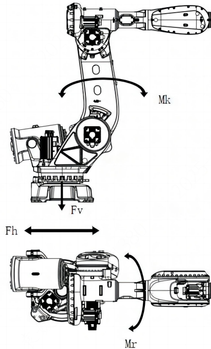
图 3-10 机器人受力图
