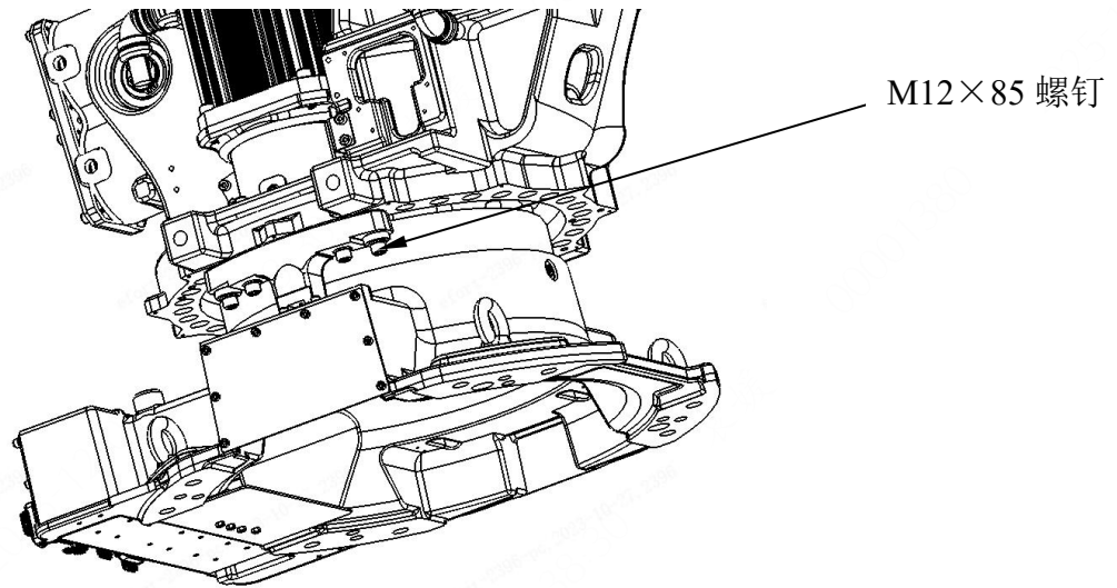
图 2-5 J1 轴可调限位图
