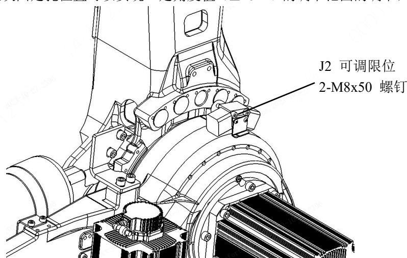
图 2-8 J2 轴可调限位图
