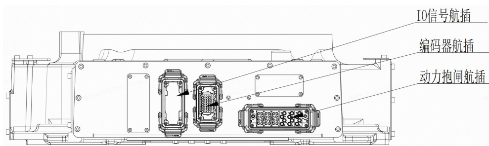
图 3-16 底座部分信号线接口
