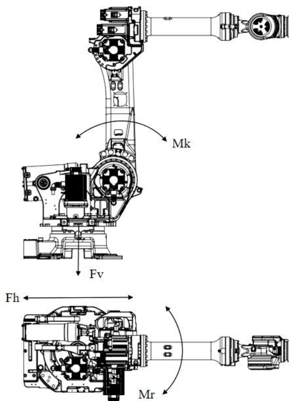
图 3-9 机器人底座受力图
