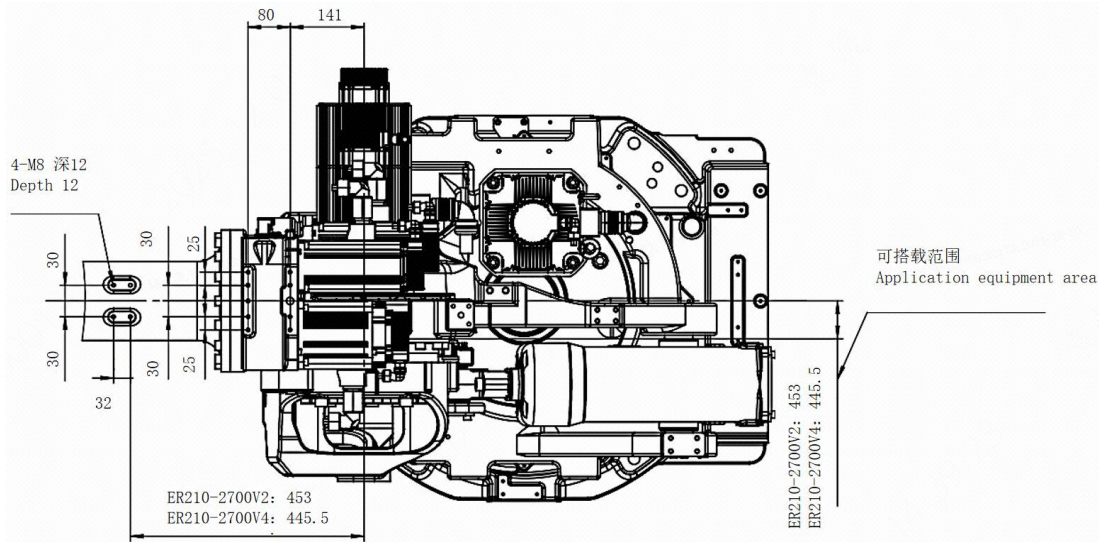
图 3-12 电机座/小臂杆上安装外部件尺寸图
