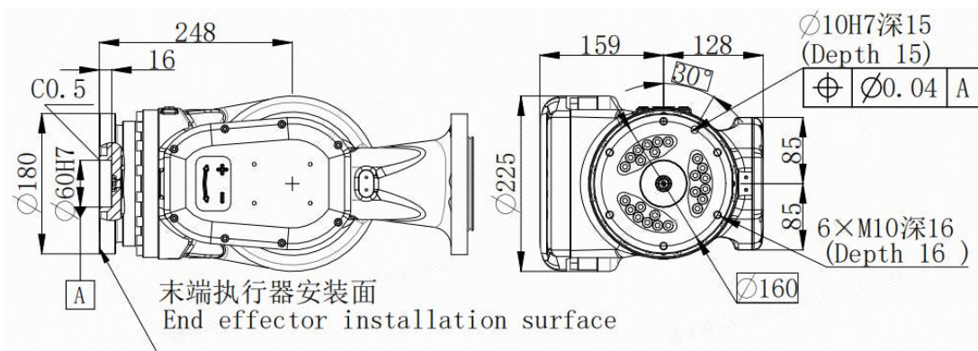
图 3-11 ER210-2700 V4 及 ER150-2700 末端负载安装法兰尺寸及末端负载安装尺寸
