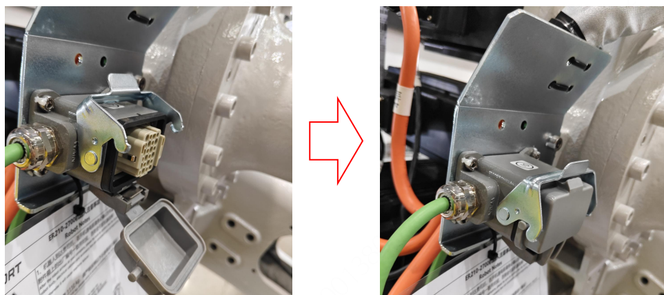
图 3-15 IO 接头安装示意图
