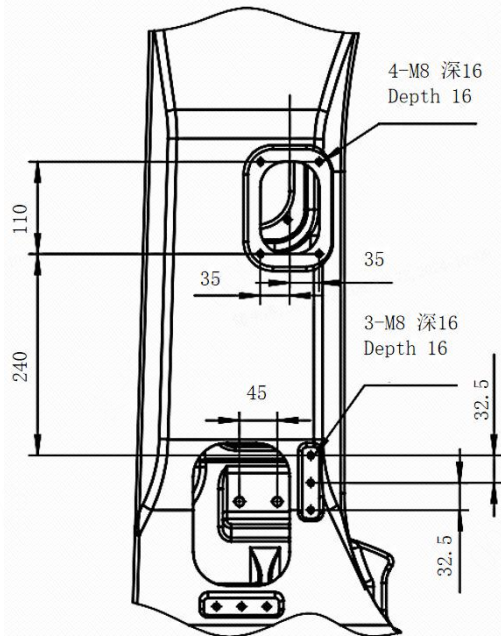
图 3-13 大臂上安装外部件尺寸图
