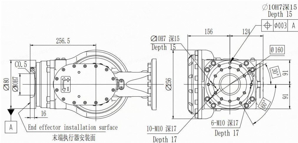
图 3-10 ER210-2700 V2 末端负载安装法兰尺寸及末端负载安装尺寸
