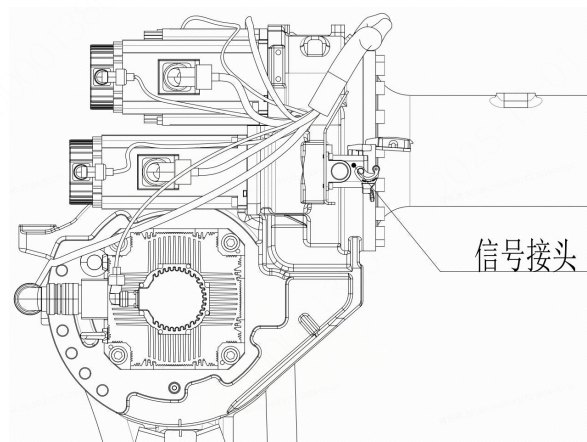
图 3-17 小臂部分信号线接口
