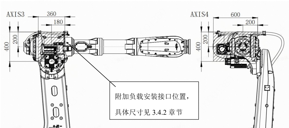
图 2-8 ER100P 下探系列上臂附加负载质心范围图
