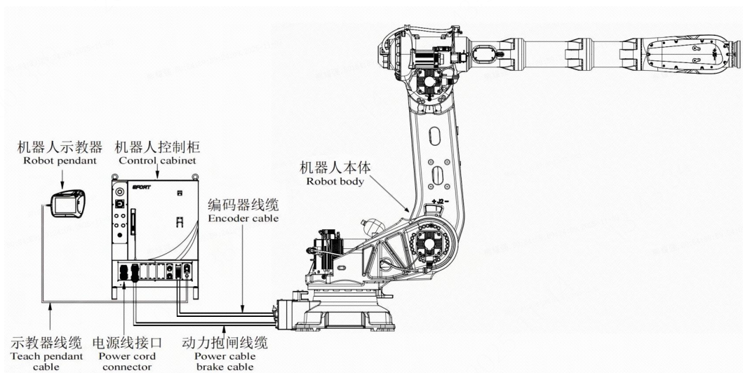
图 2-1 工业机器人系统构成
