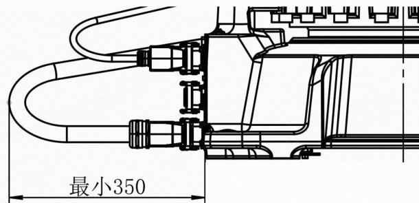
图 3-6 底座线缆后侧出线最小弯折尺寸
