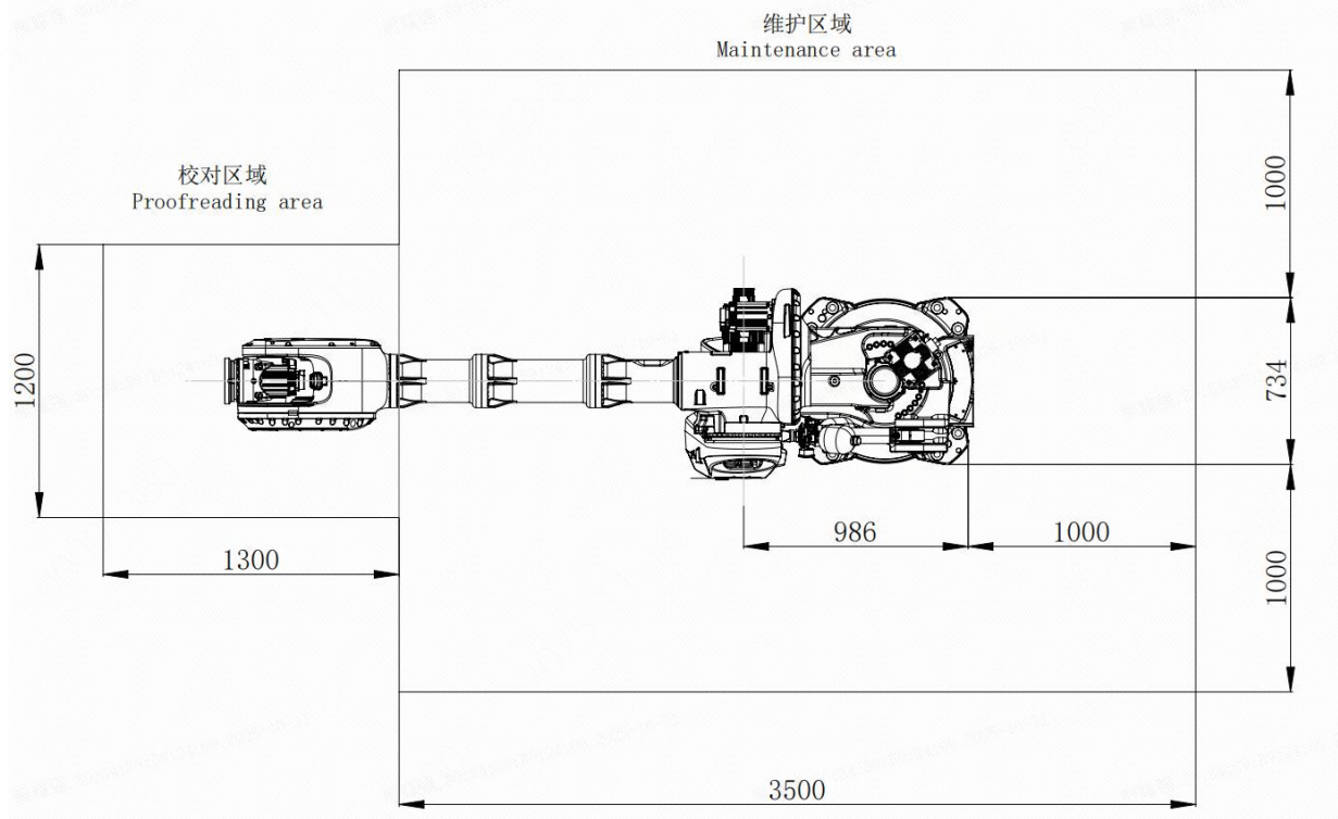
图 4-2 维护及使用区域
