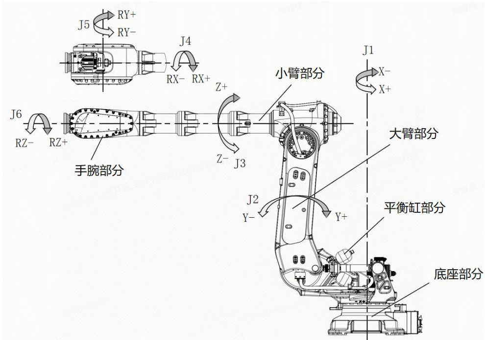
图 2-3 ER100P 下探系列机械本体组成部分
