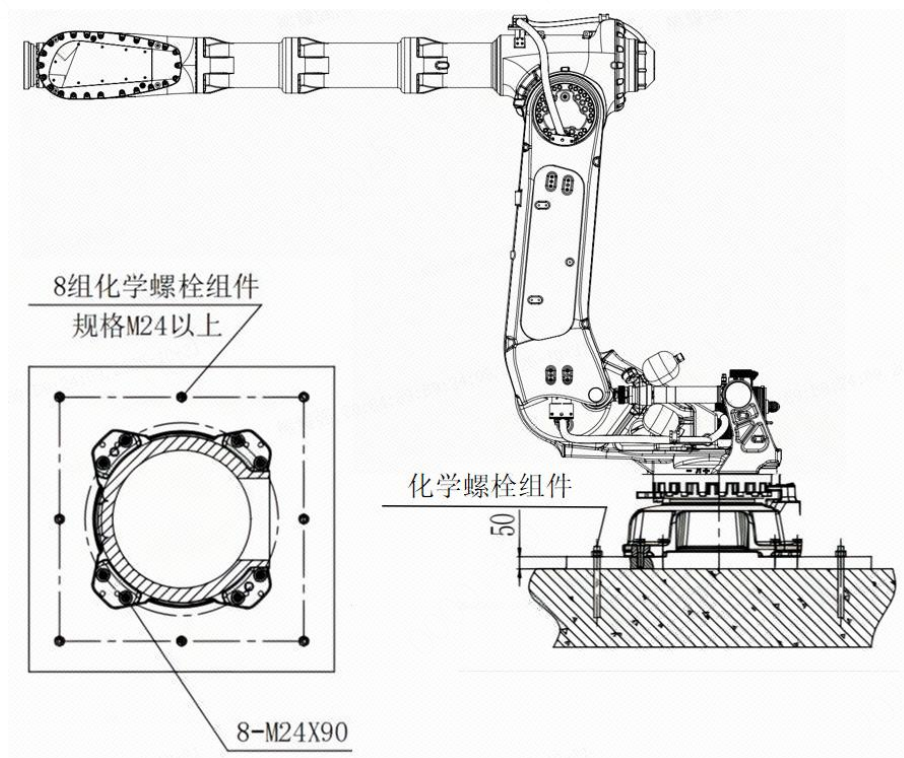
图 3-9 机器人安装举例
