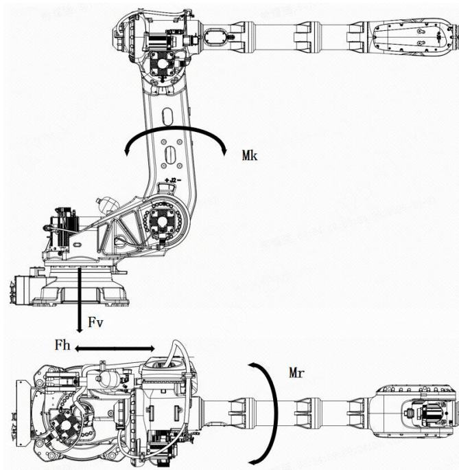
图 3-10 机器人受力图
