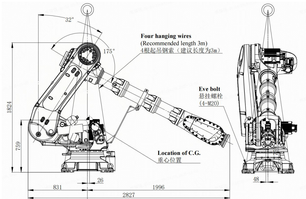
图 3-3 吊装搬运示意图
