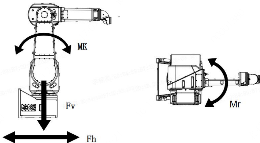
图 3-10 机器人受力图
