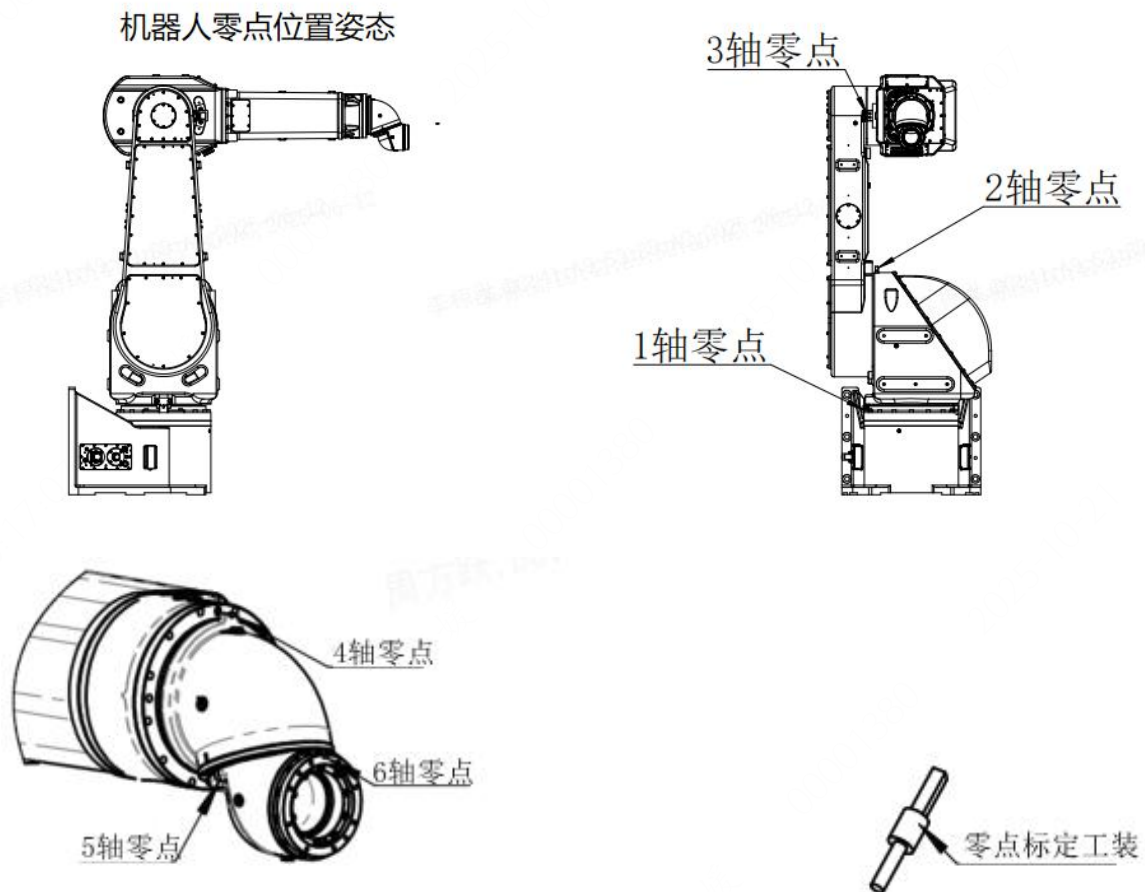
图 4-6 机器人零点位置图
