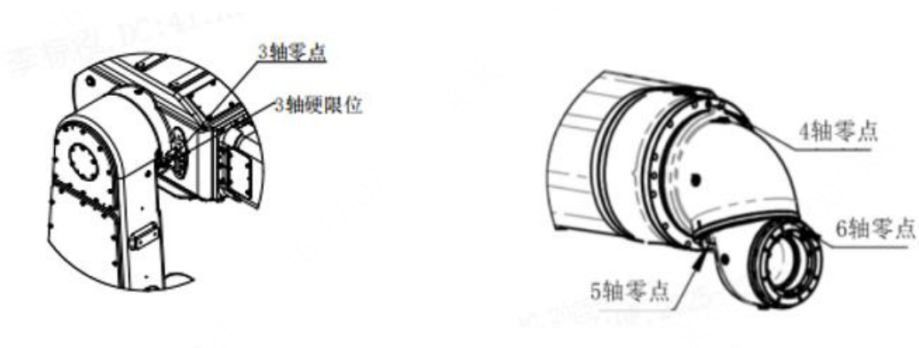
图 2-4 机械硬限位位置及零标位置
