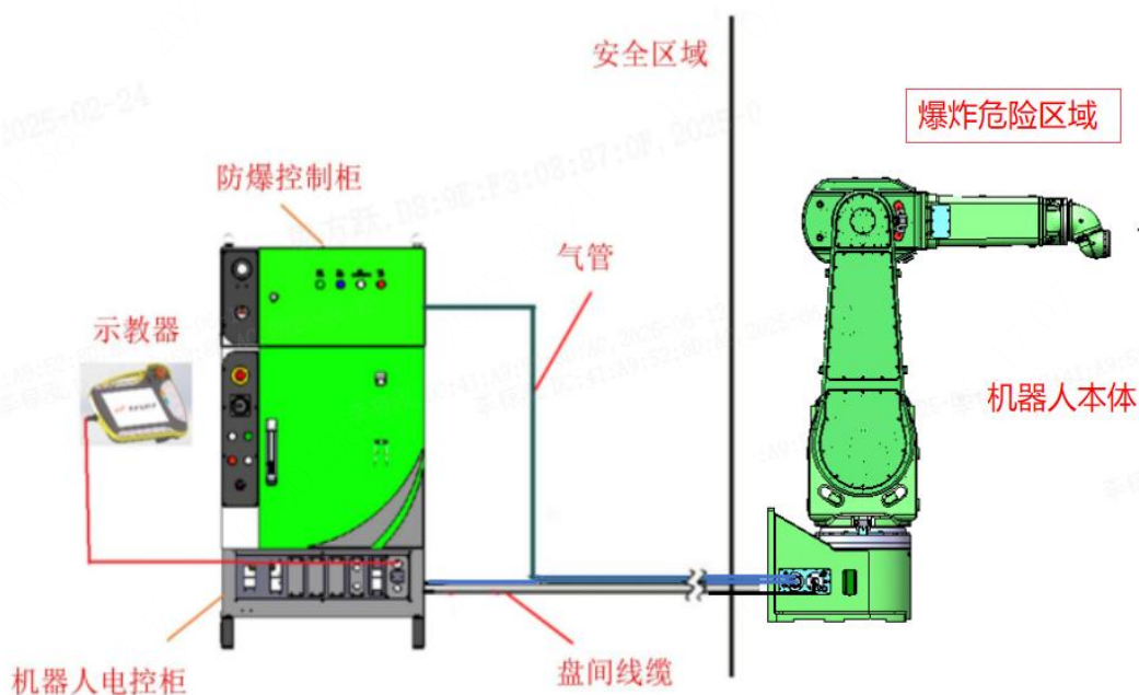
图 2-1 工业机器人系统构成
