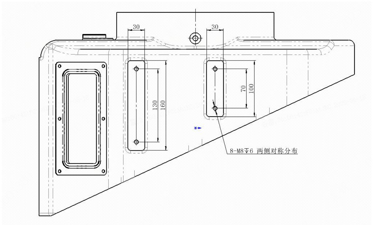
(b) 电机座
