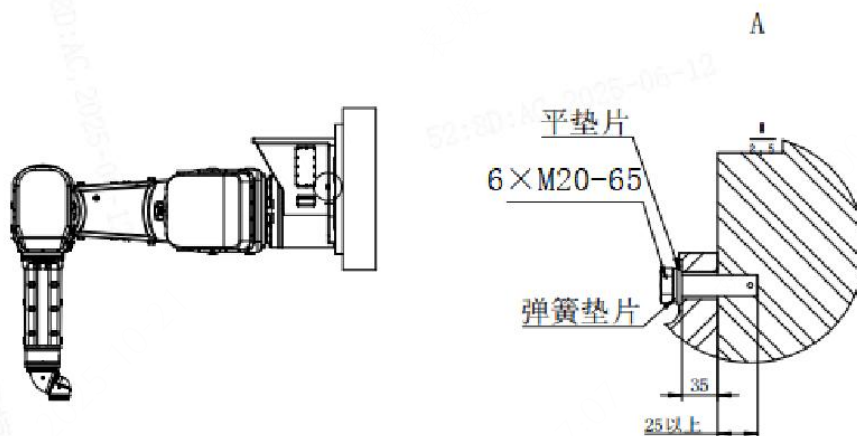
图 3-8 壁挂安装
