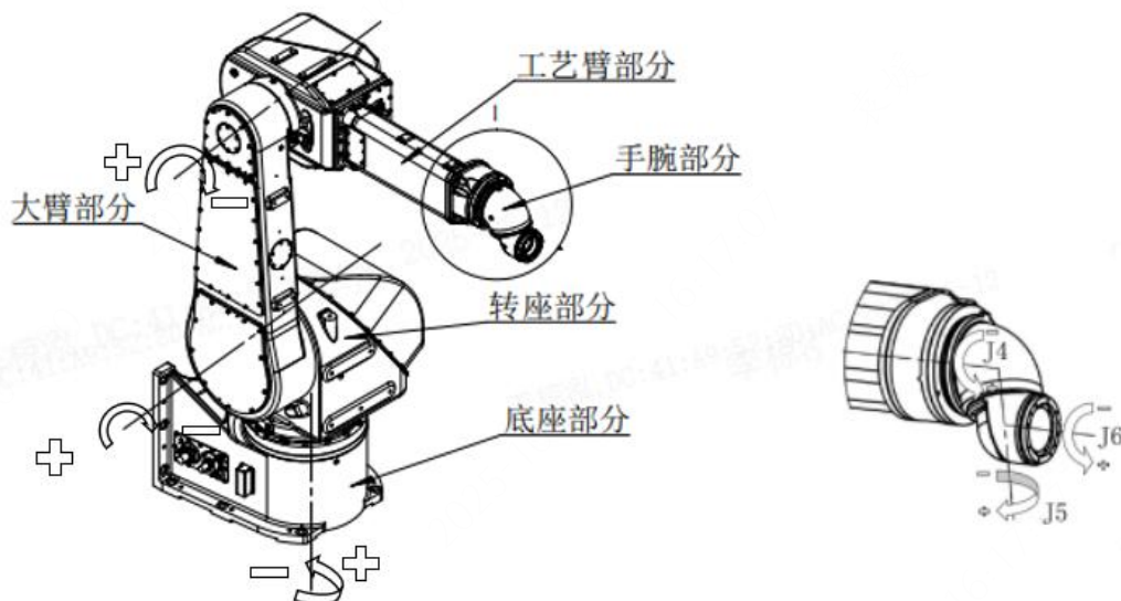
图 2-3 机械本体组成部分
