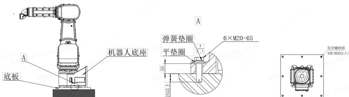
图 3-7 机器人安装举例
