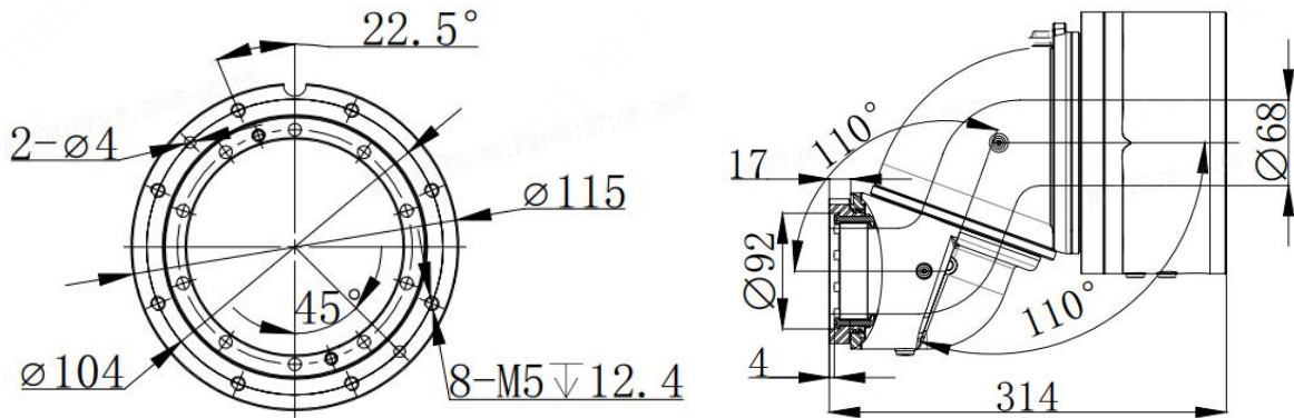
图 3-11 末端负载安装法兰尺寸
