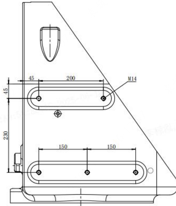
(d) 转座
