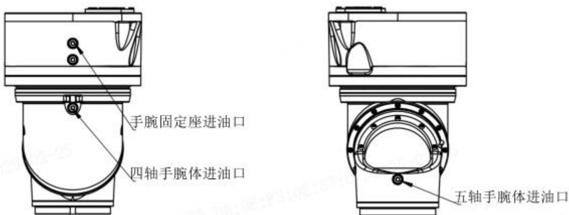
图 4-1 机器人注油口和排气口分布图
