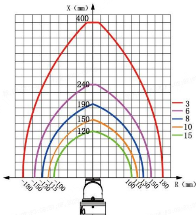
图 2-6 GR6150-2000/2200/2500/2900 手腕轴转矩图
