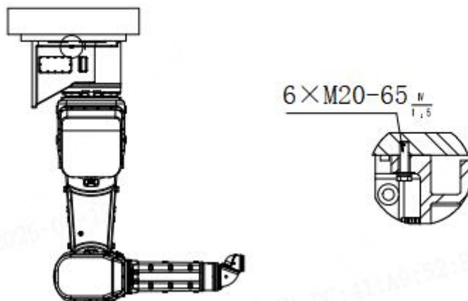
图 3-9 倒挂安装
