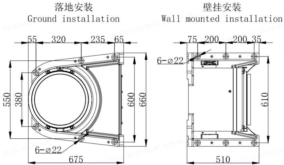
图 3-3 机器人底座尺寸
