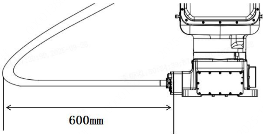
图 3-4 底座线缆后测出线弯折尺寸
