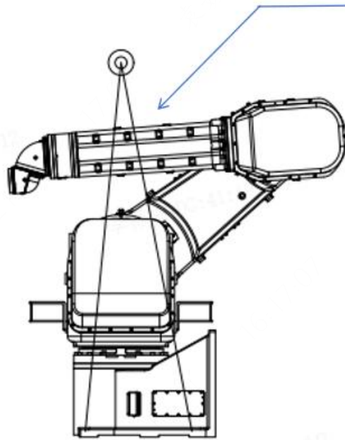
图 3-1 吊装搬运示意图
