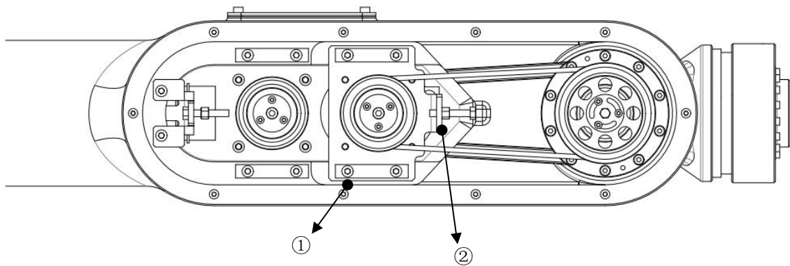
注：①固定螺钉，4个 M5×16；②调距螺钉，1个 M5×35
