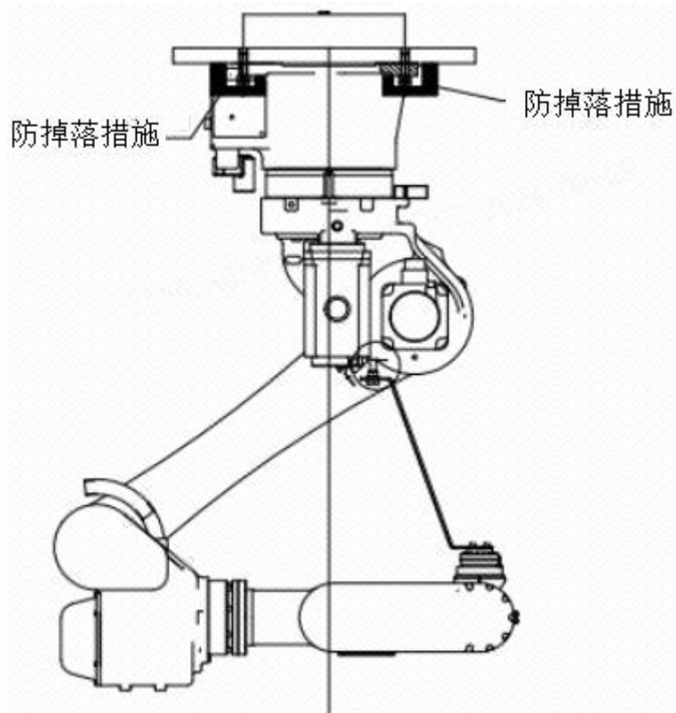
图 3-8 倒挂安装示例
