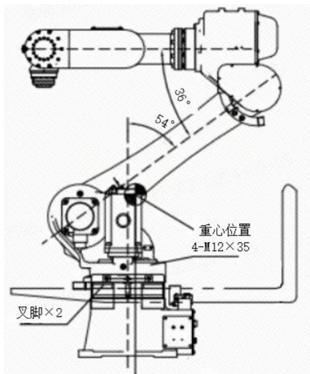
图 3-4 ER20-1700 叉车搬运示意图
