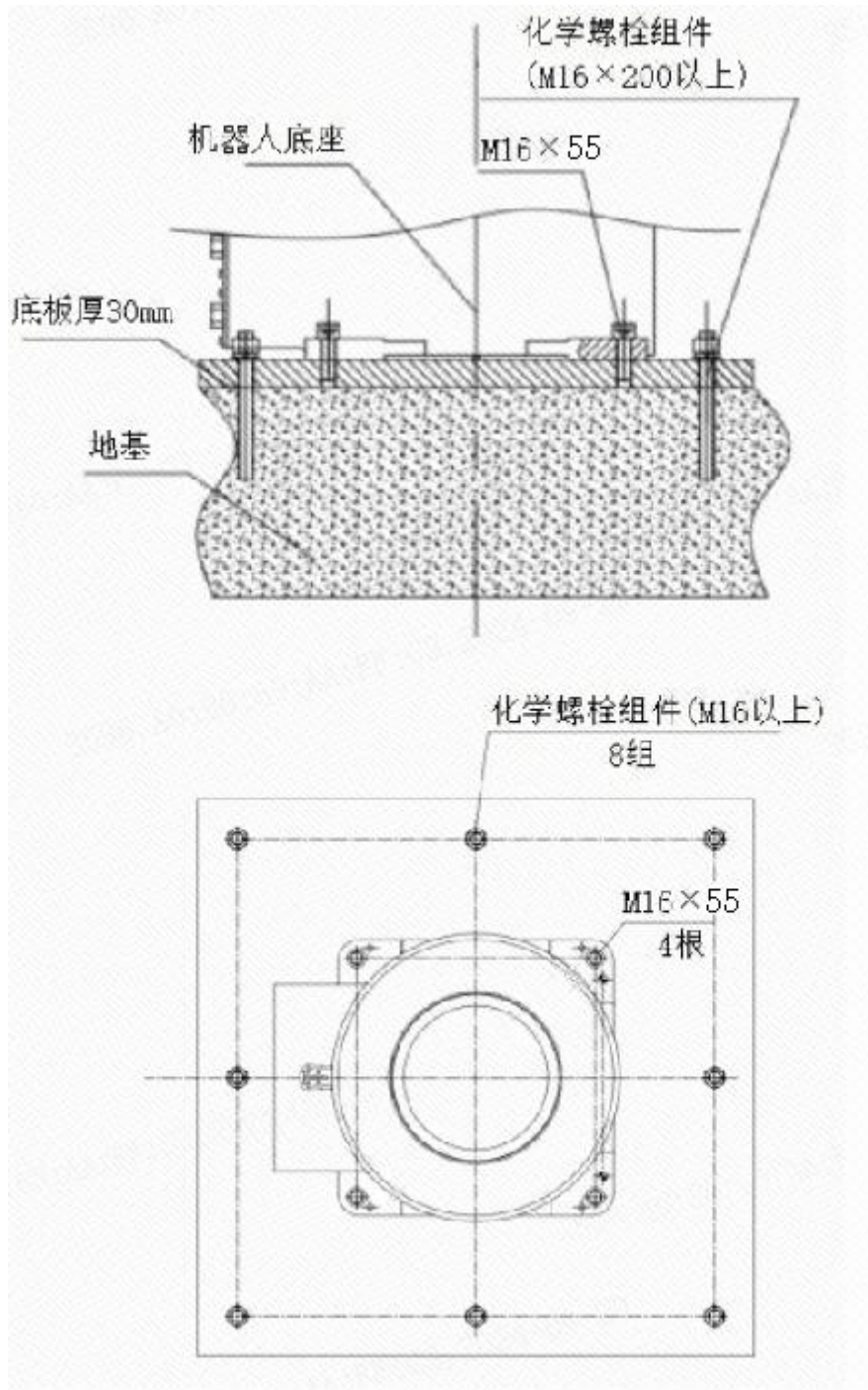
图 3-7 机器人安装举例
