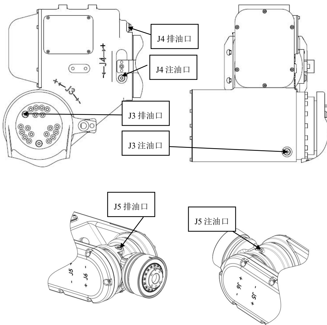
图 4-1 机器人注油口和排气口分布图
