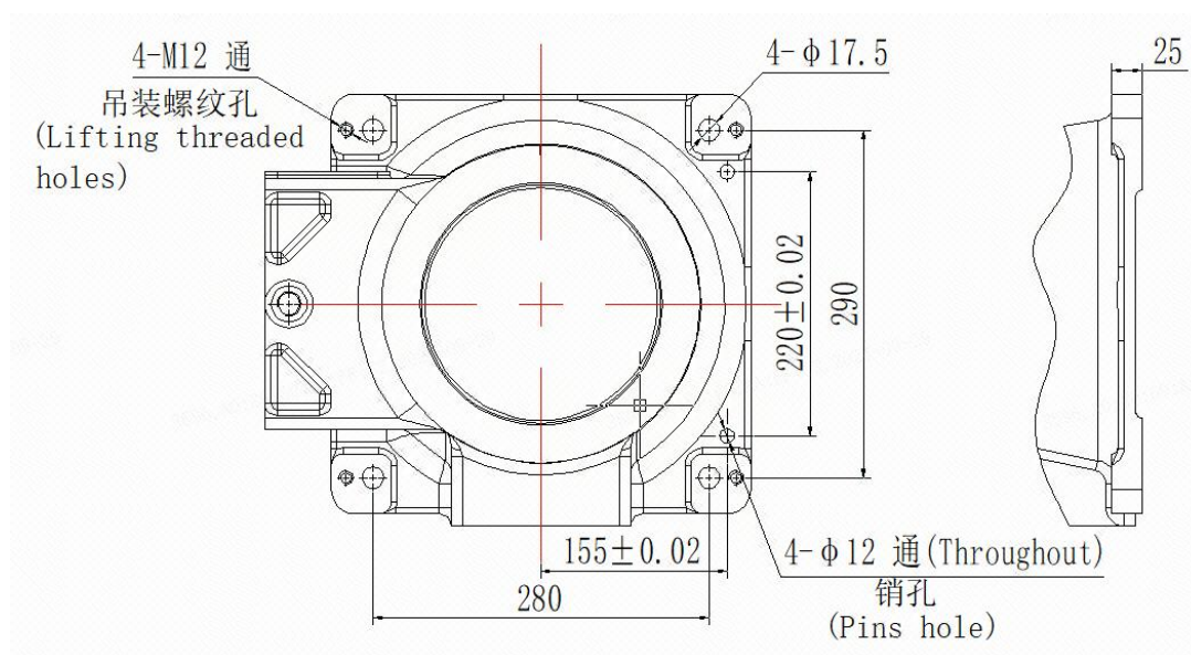
图 3-5 机器人底座尺寸
