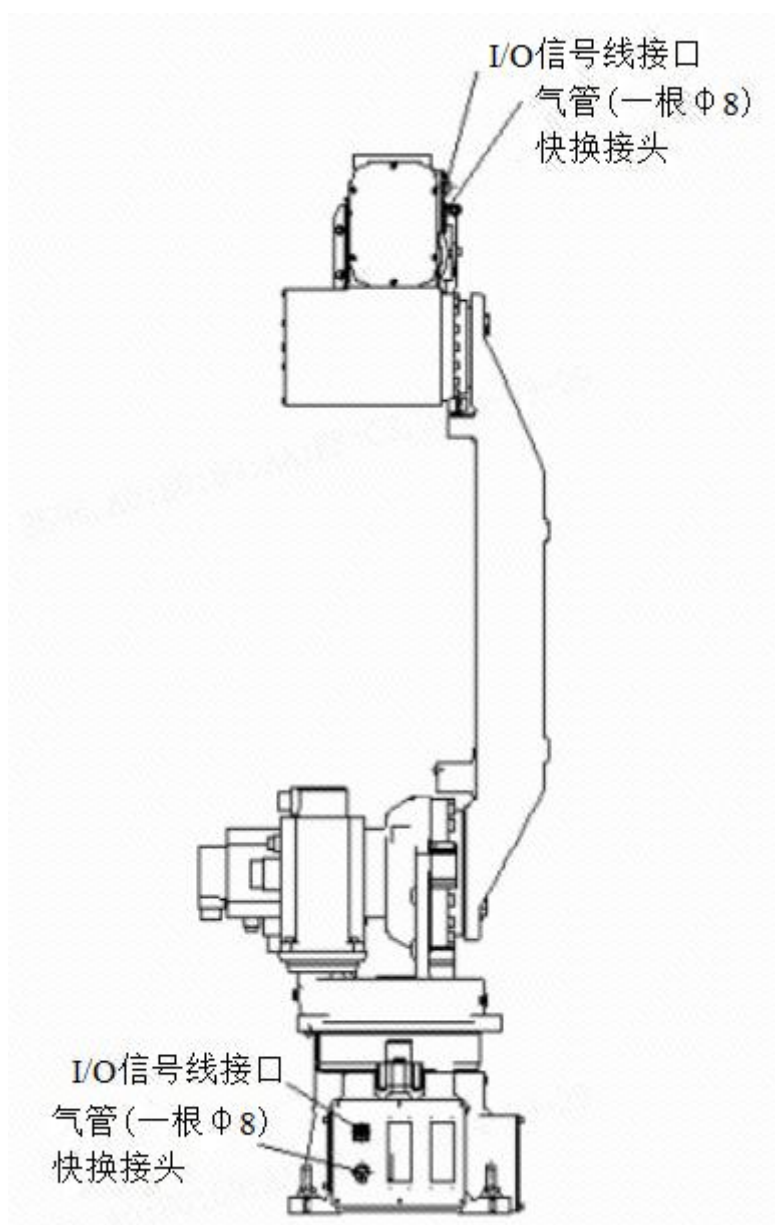
图 3-12 外接气管和信号线
