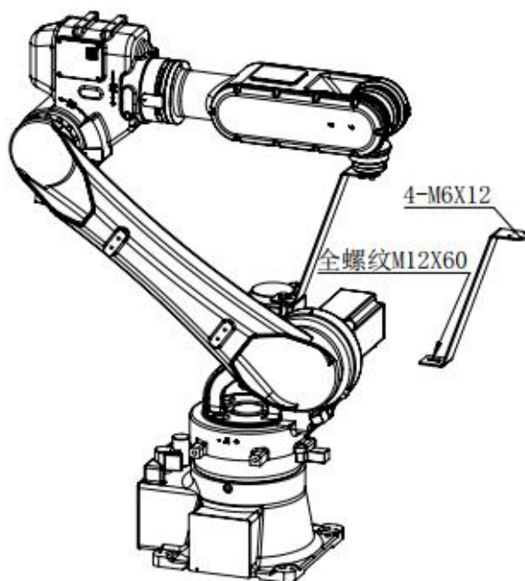
图 3-1 打包固定支架安装示意图
