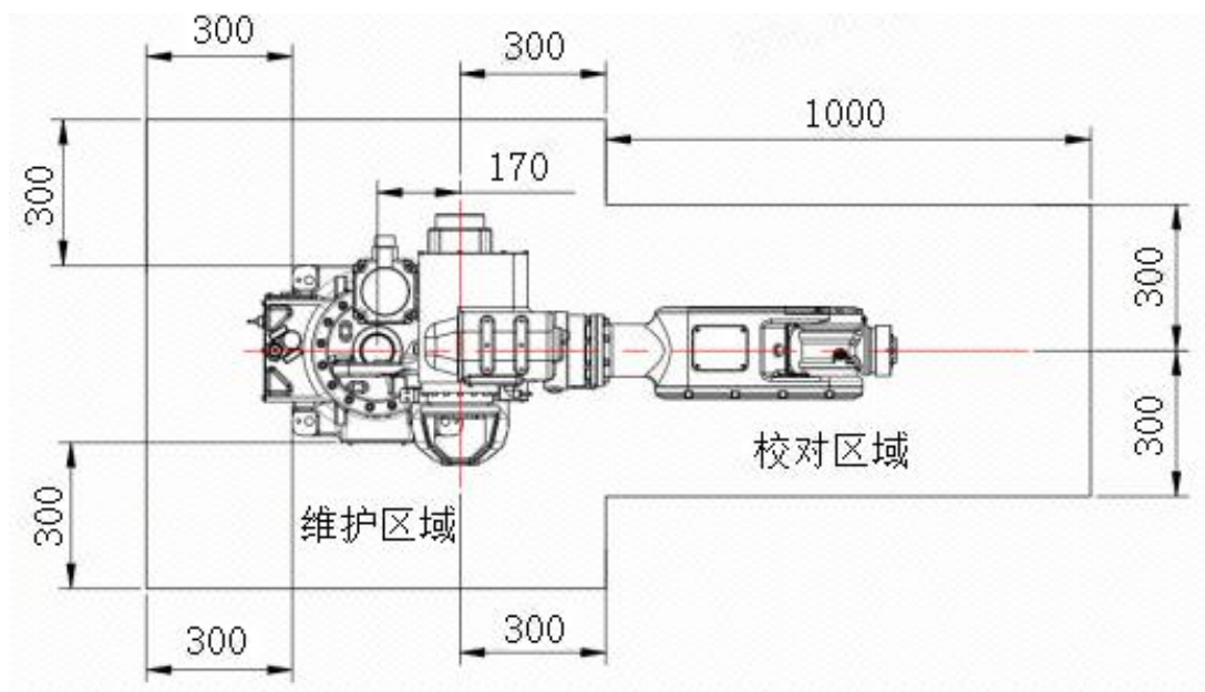
图 4-4 维护及使用区域
