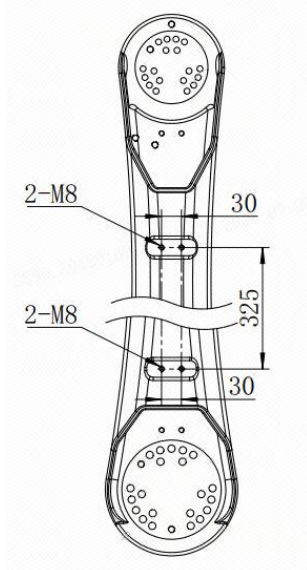
图 3-10 大臂上安装外部件尺寸图
