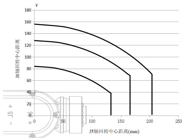
图 2-6 ER20-1700 手腕轴转矩图
