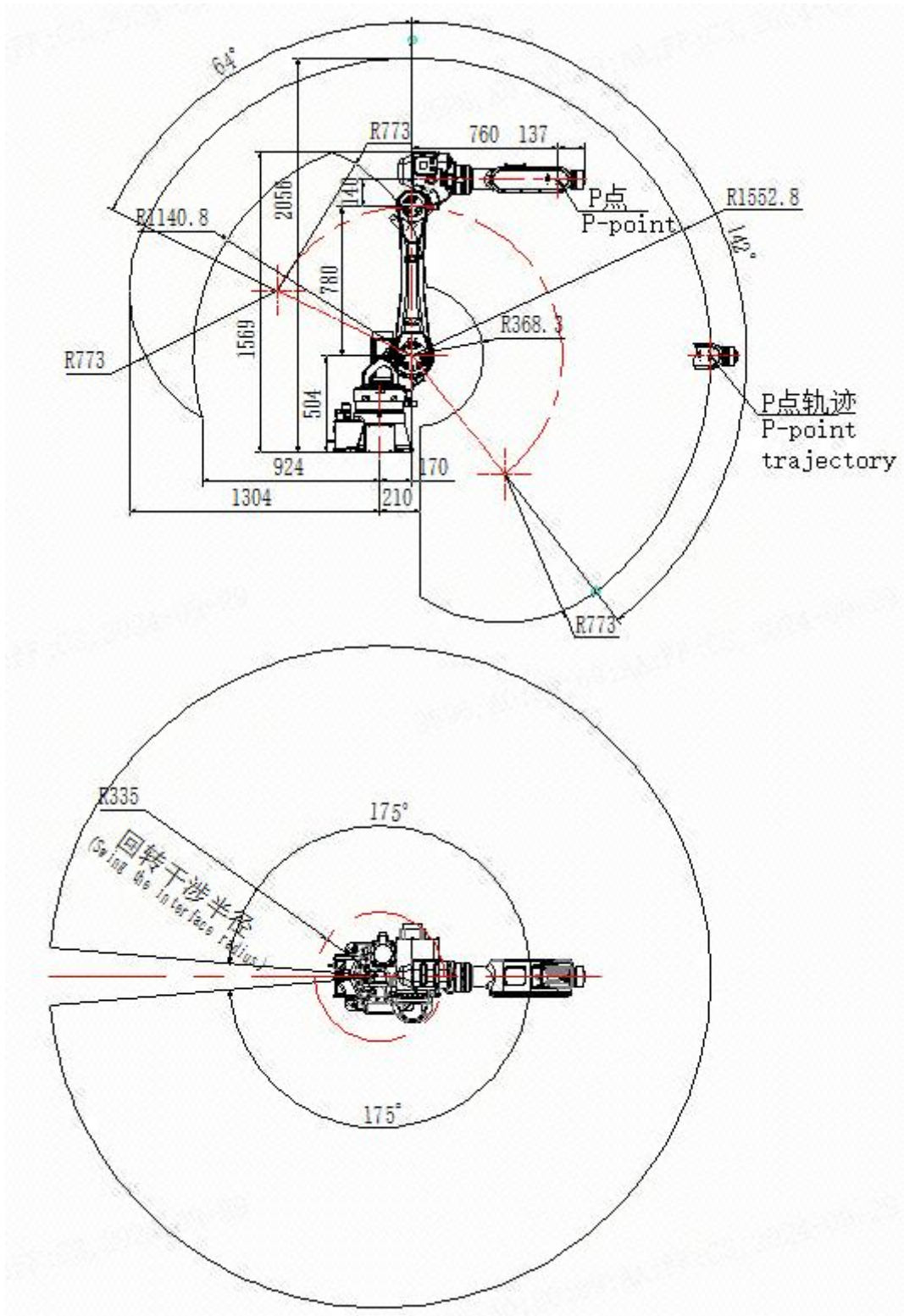
图 2-5 ER20-1700 机器人工作空间图
