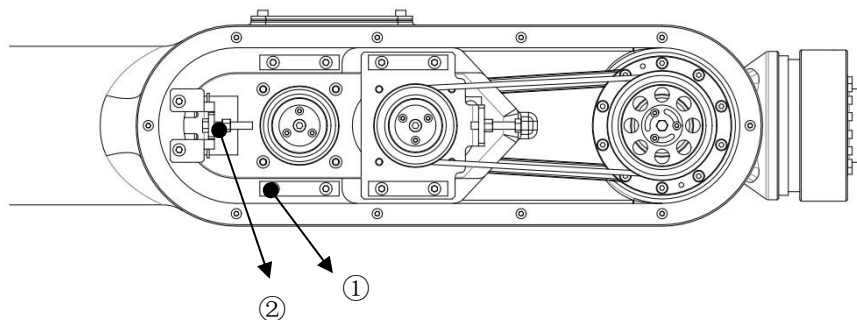
图 4-2 ER20-1700 机器人 J5 轴同步带结构图
