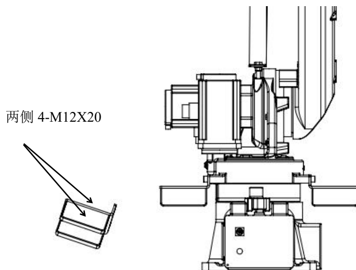
图 3-2 叉脚安装示意图
