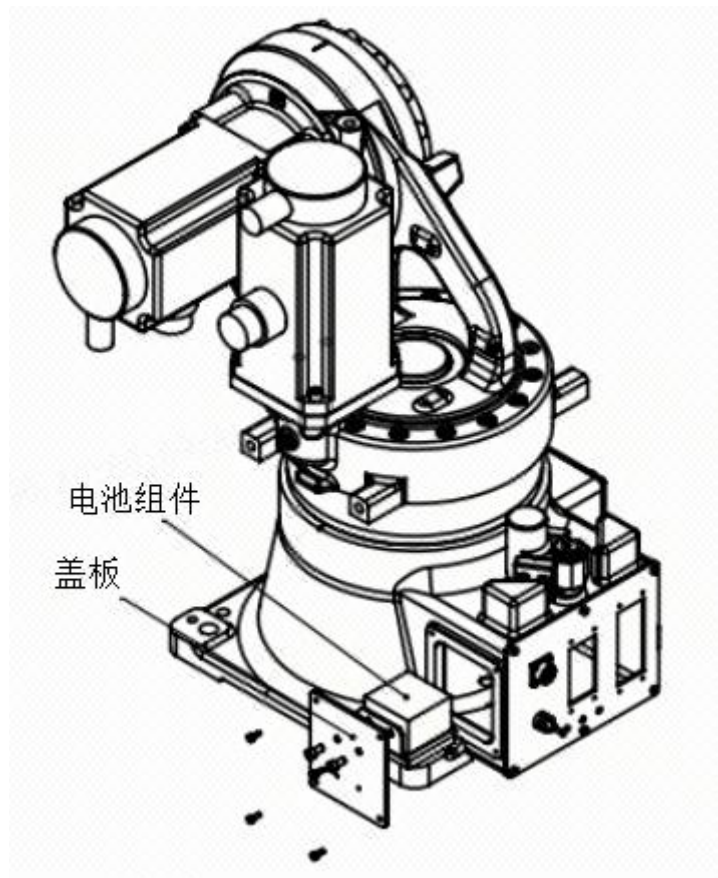
图 4-6 机器人电池组位置图
