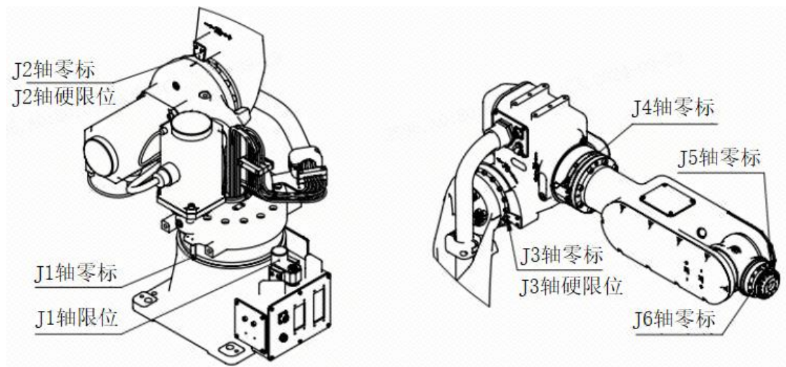
图 2-4 机械硬限位位置及零标位置
