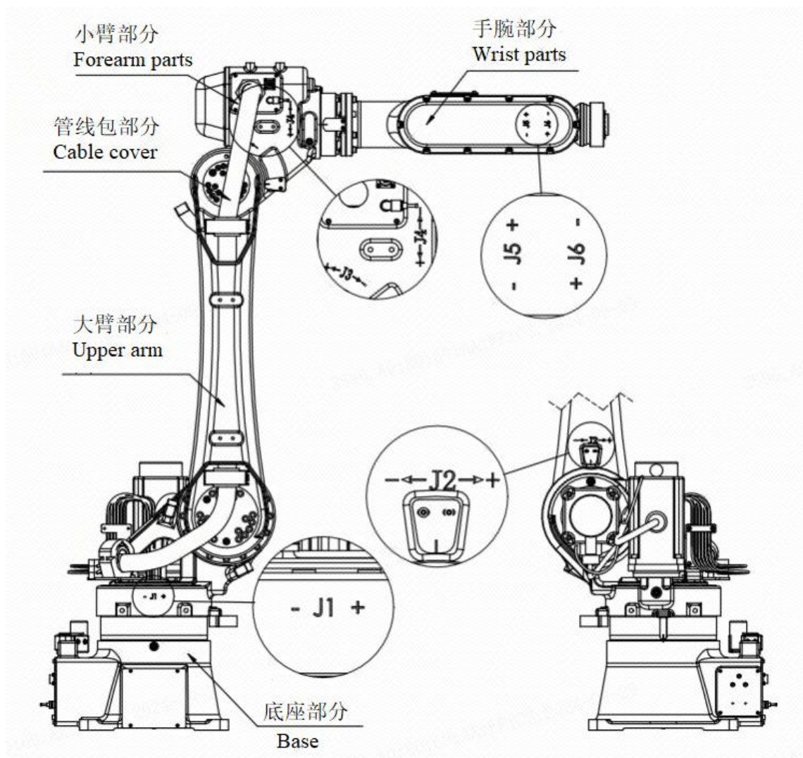
图 2-3 ER20-1700 机械本体组成部分
