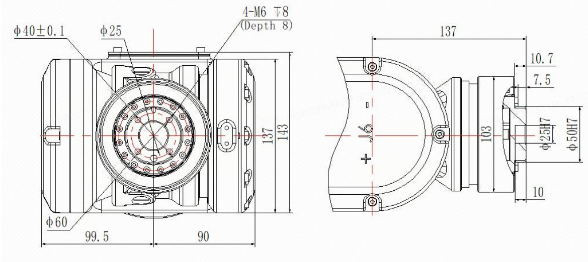
图 3-9 末端负载安装法兰尺寸
