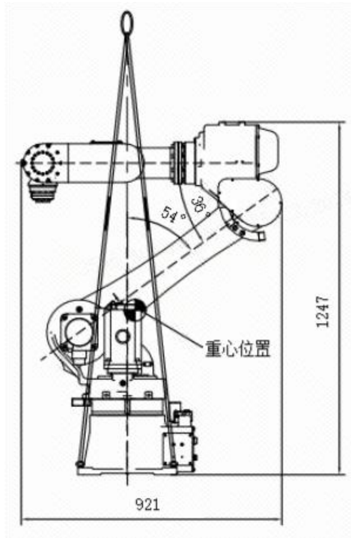
图 3-3 ER20-1700 吊装搬运示意图
