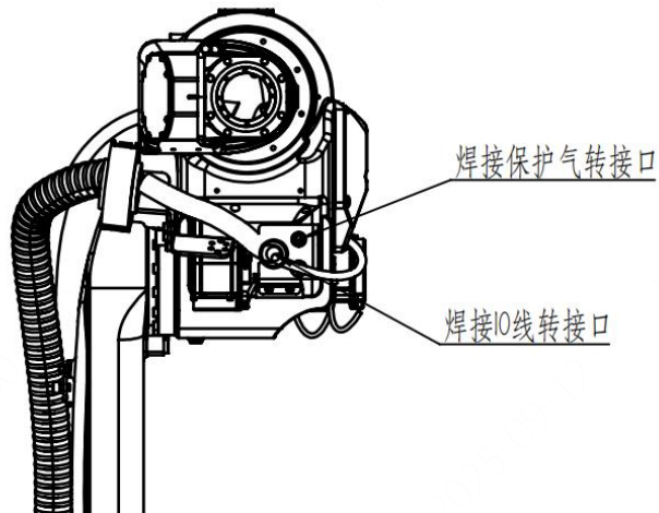
图 3-15 电机座部分气路及信号线接口
