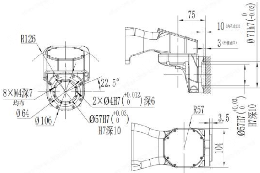
图 3-11 末端负载安装法兰尺寸
