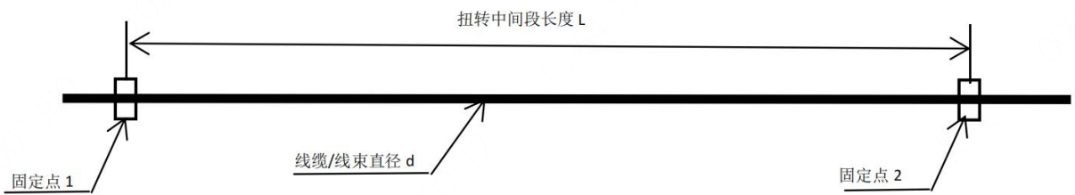
图 3-6 线缆/线束扭转距离
