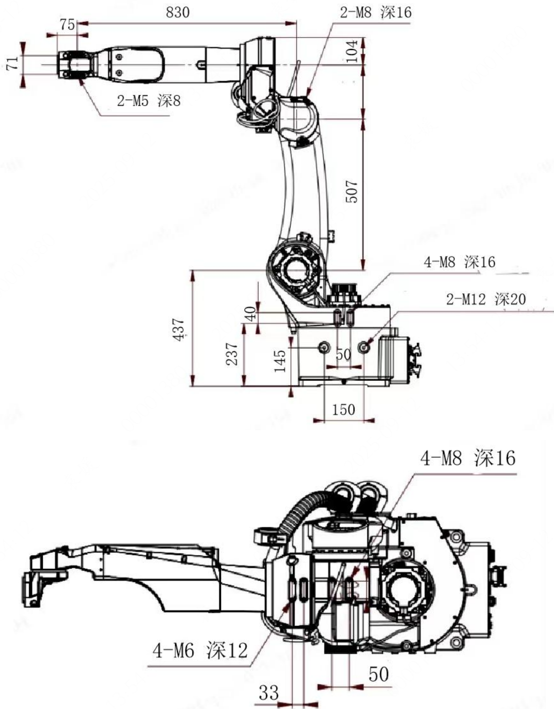
图 3-12 外围安装尺寸图
