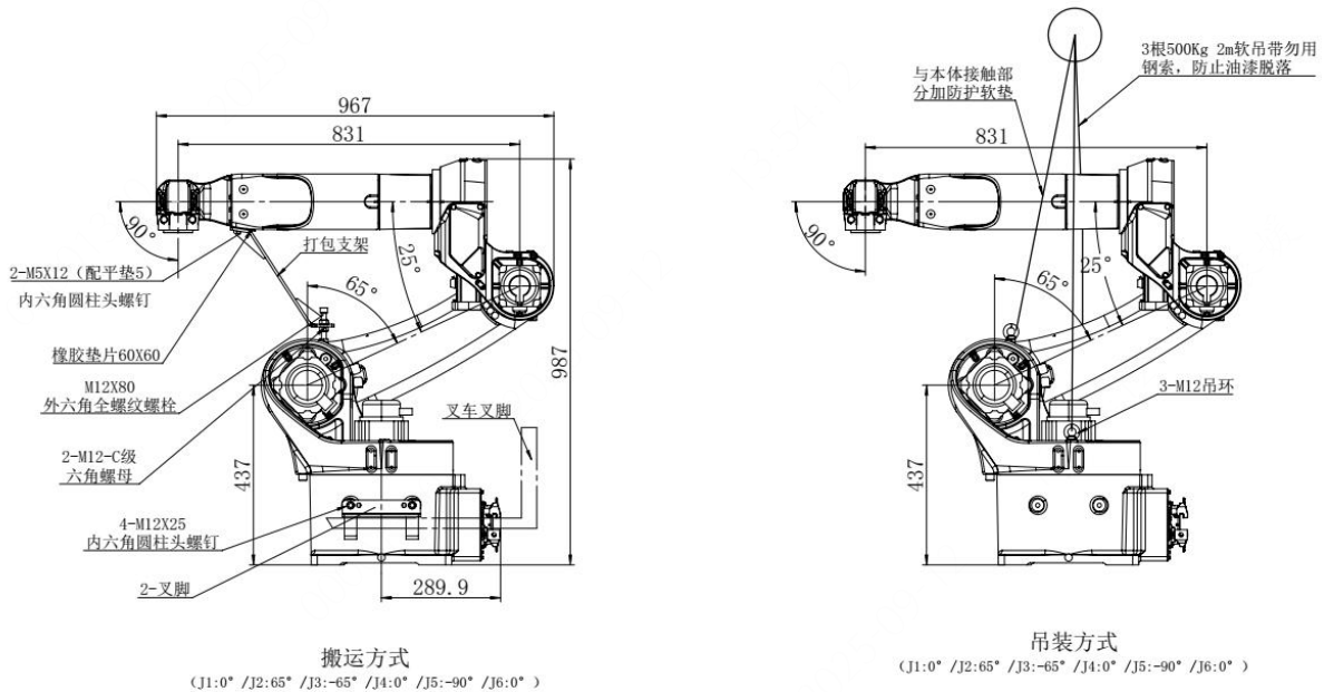
图 3-3 转运示意图
