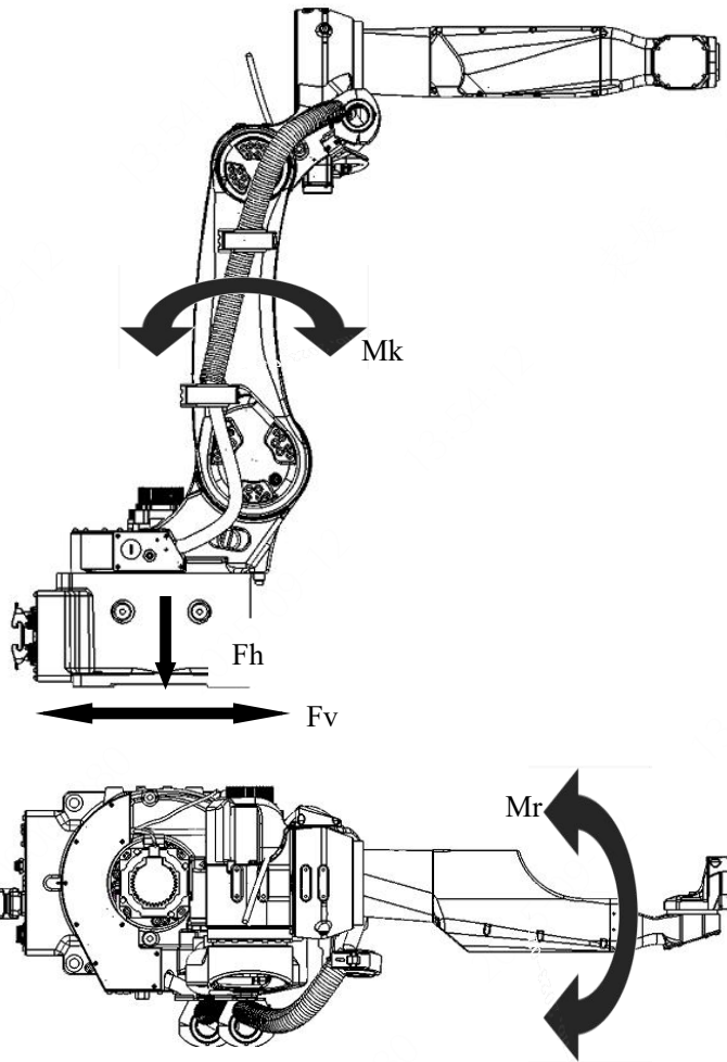
图 3-10 机器人受力图
