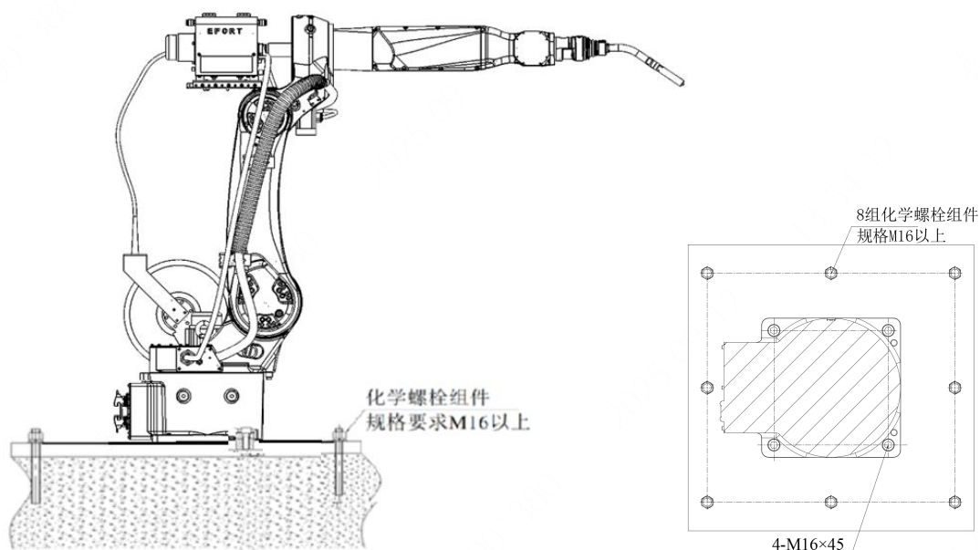
图 3-8 机器人安装举例
