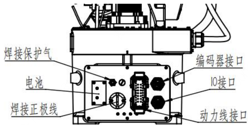
图 3-14 底座部分气路及信号线接口
