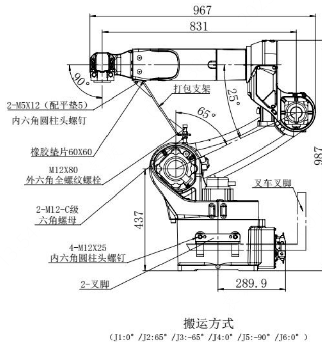
图 3-1 打包固定支架安装示意图
