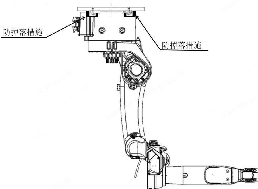
图 3-9 机器人倒装案例
