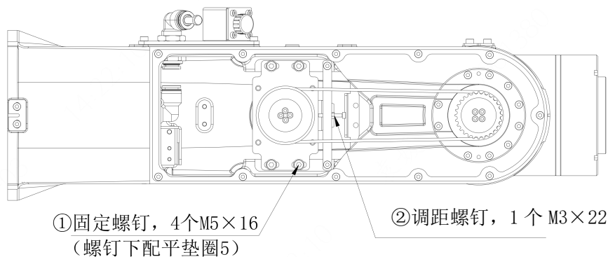
图 4-2 ER15-1400 机器人 J5 轴同步带结构图
