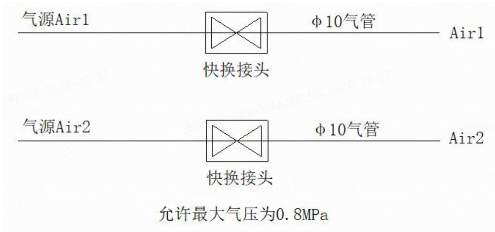
图 3-19 标准型气路原理图（标准）
