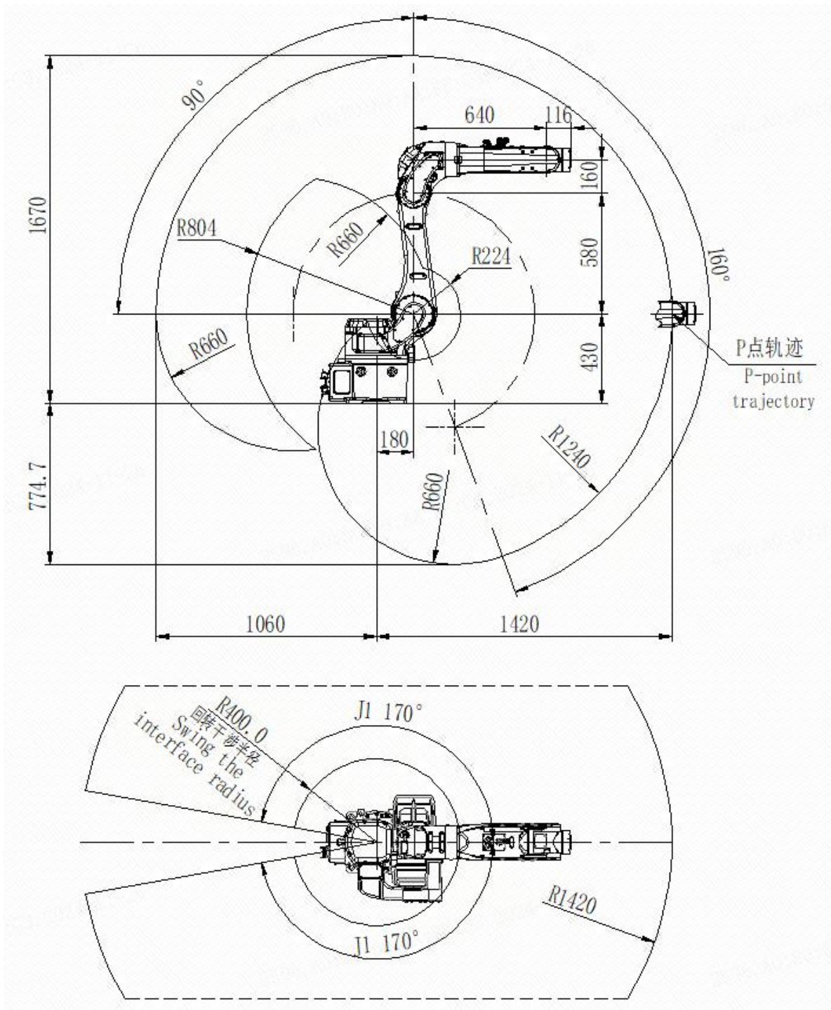
图 2-6 机器人工作空间图
