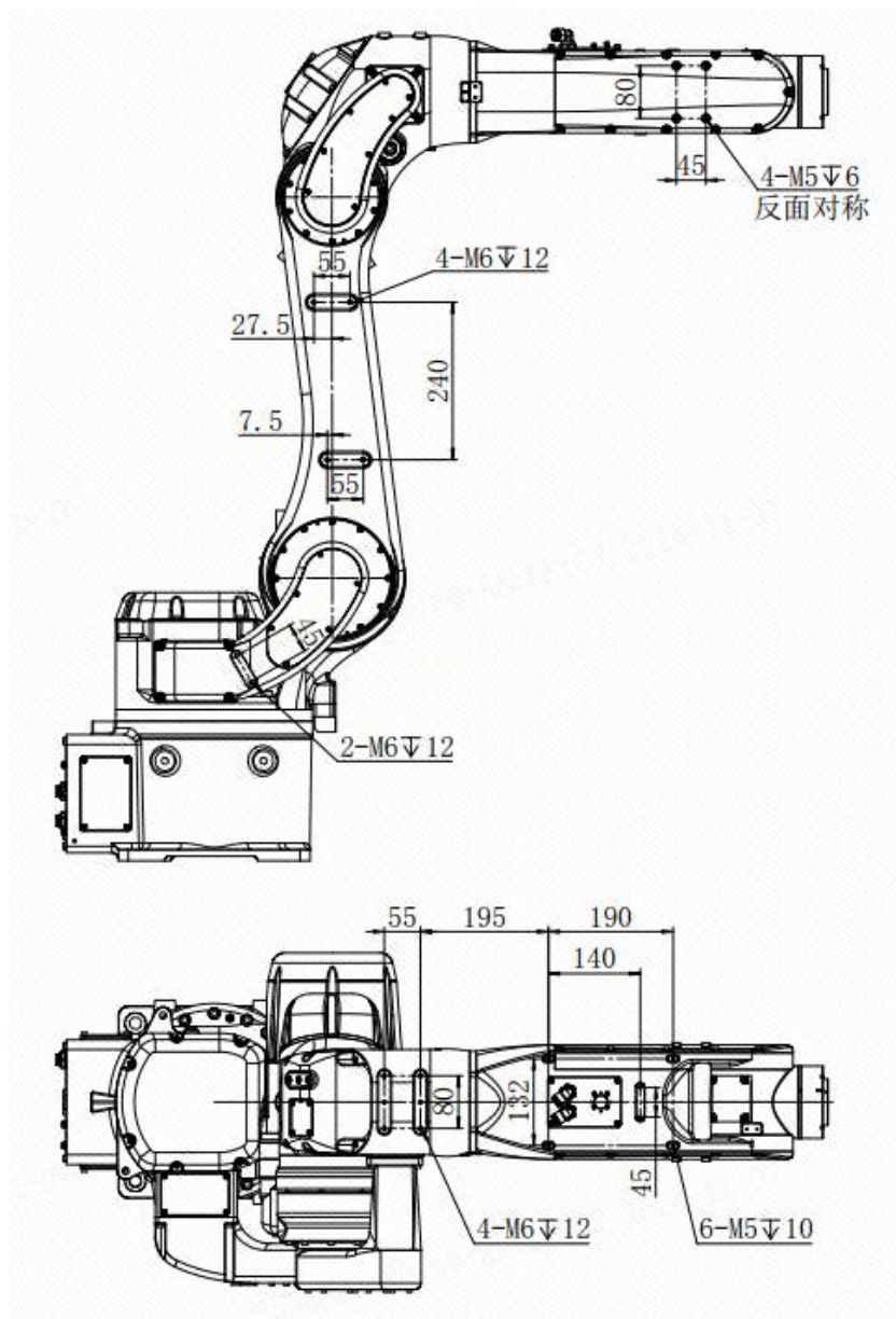
图 3-13 外围安装尺寸图
