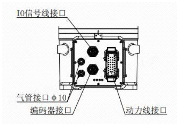
图 3-20 底座部分气路及信号线接口
