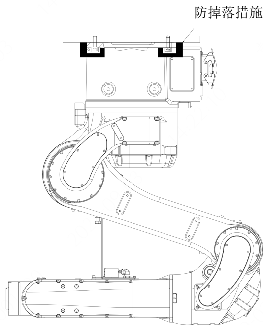
图 3-10 倒挂安装
