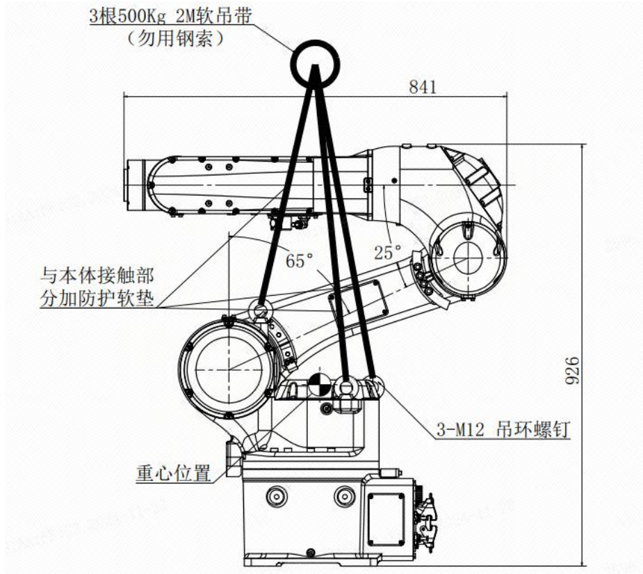
图 3-3 吊装搬运示意图
