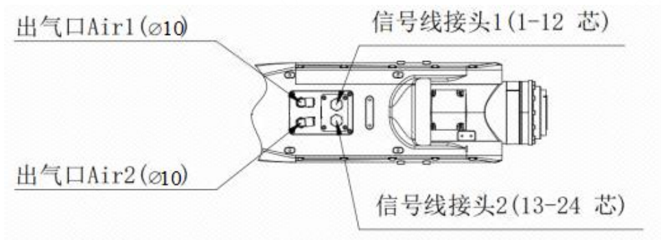
图 3-21 小臂部分气路及信号线接口
