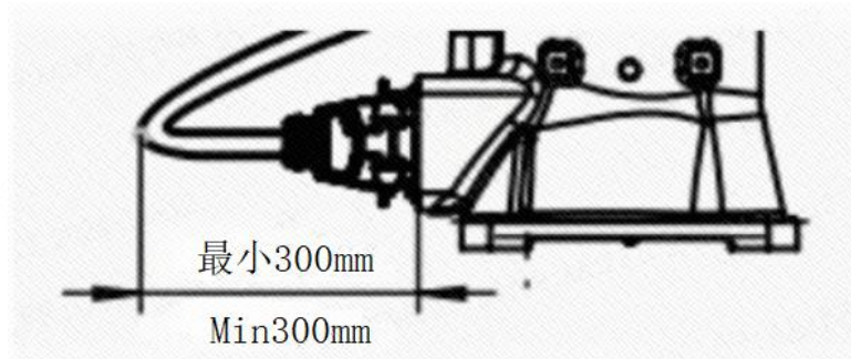
图 3-6 底座线缆后侧出线最小弯折尺寸
