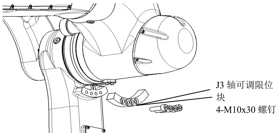
图 2-5 J3 轴可调限位图
