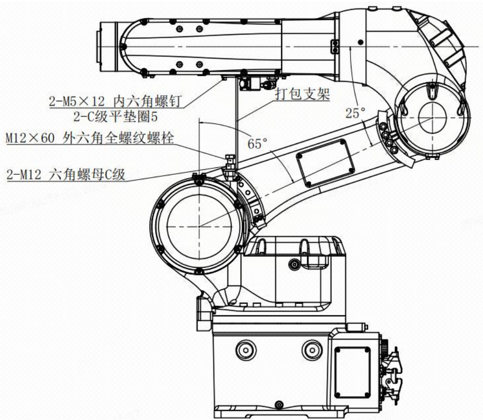
图 3-1 打包固定支架安装示意图
