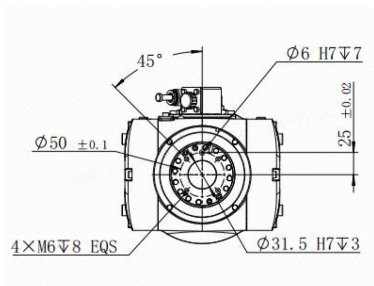
图 3-12 末端负载安装法兰尺寸
