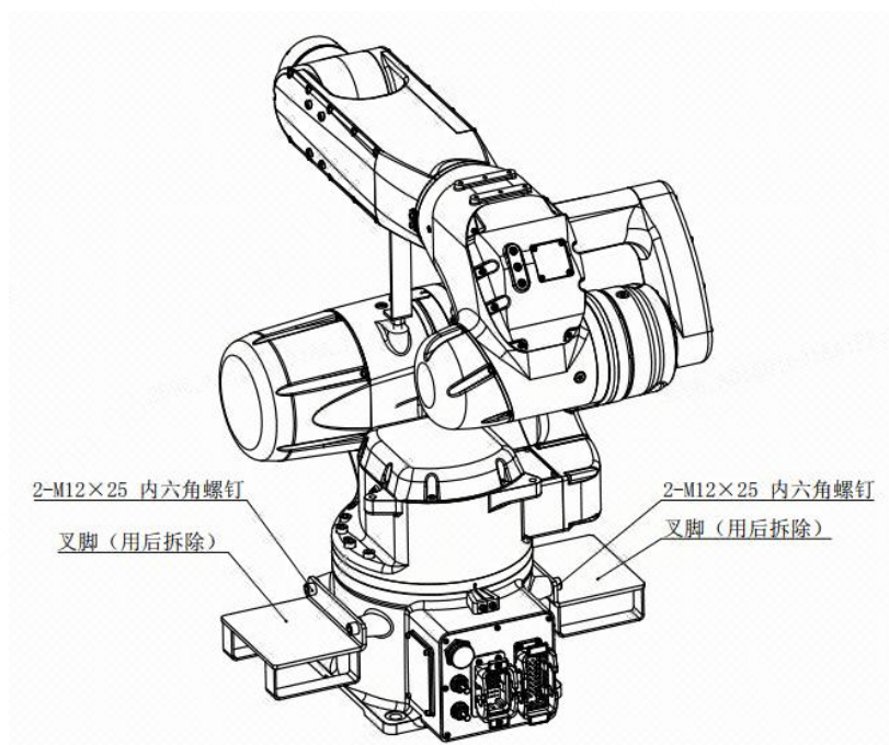
图 3-2 叉脚安装示意图
