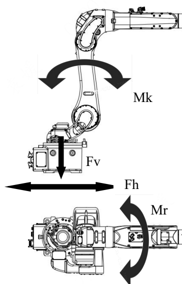
图 3-11 机器人受力图
