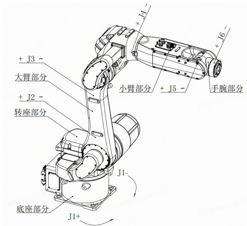
图 2-3 ER15-1400 机械本体组成部分
