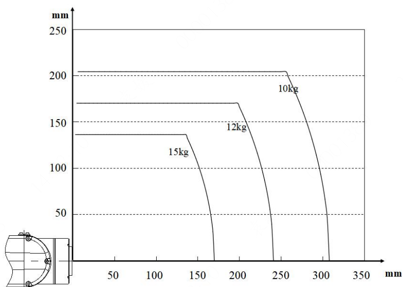
图 2-7 ER15-1400 手腕轴转矩图
