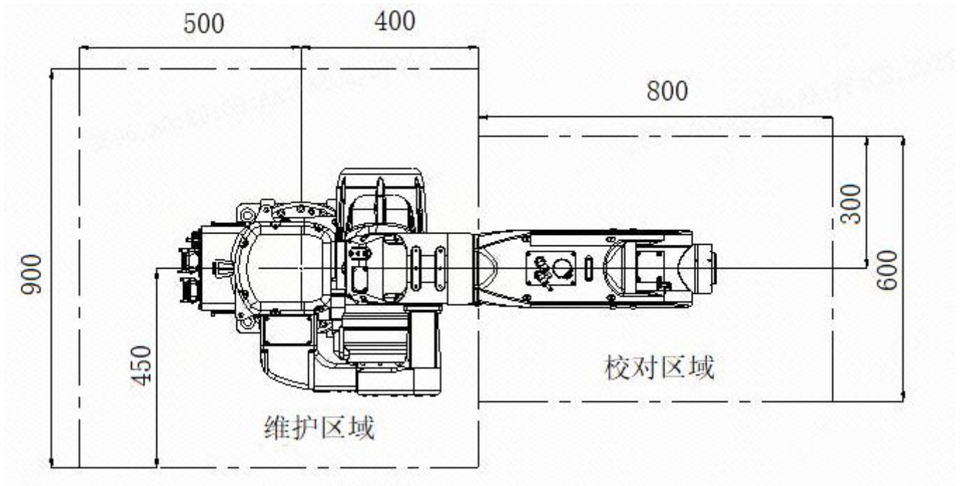
图 4-3 维护及使用区域
