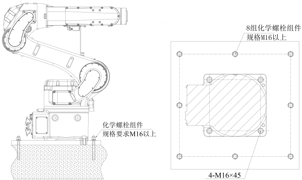
图 3-9 机器人安装举例
