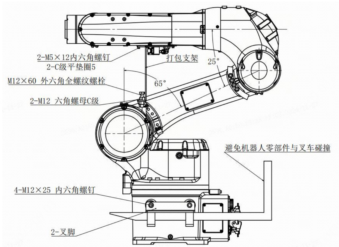
图 3-4 叉车搬运示意图
