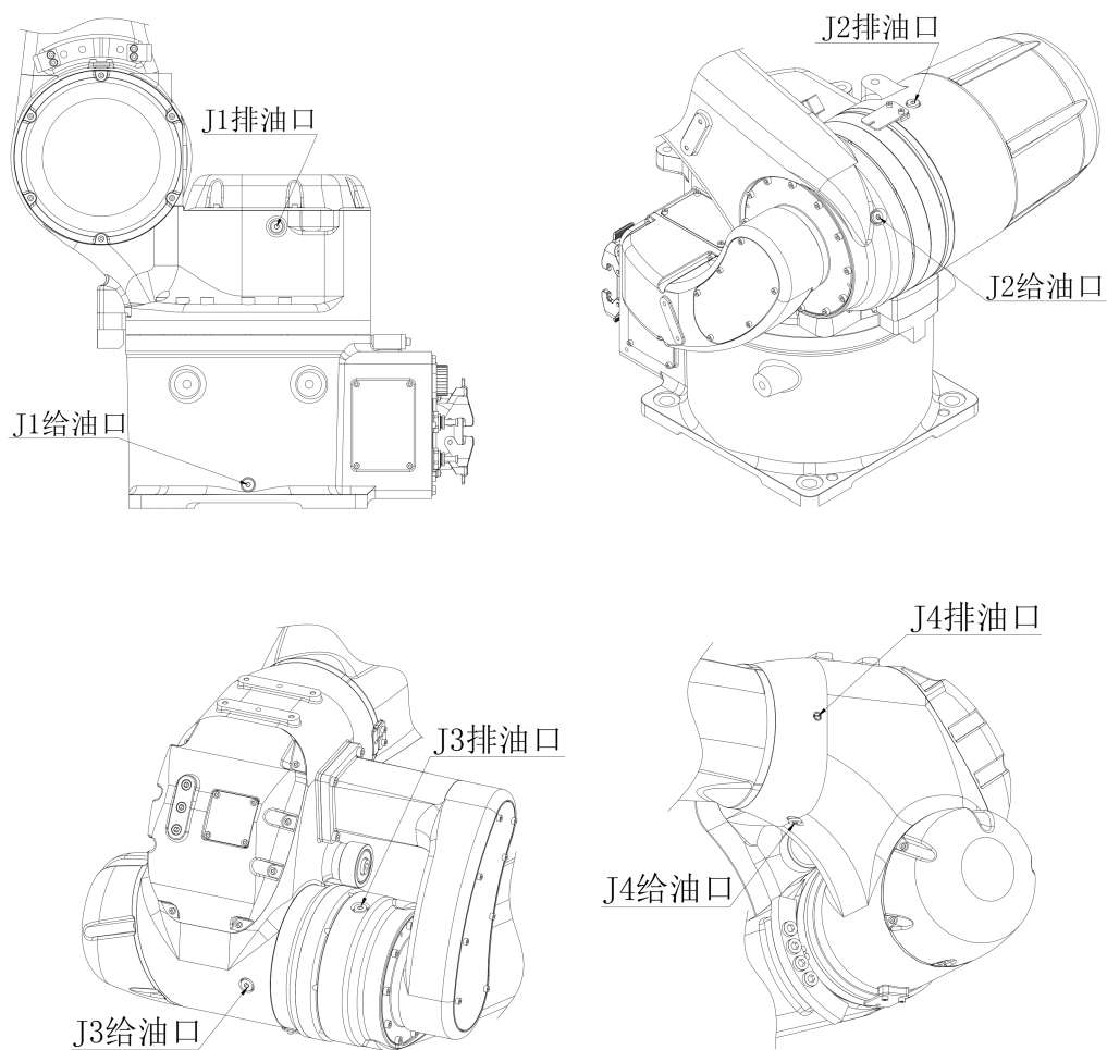
图 4-1 机器人进油口和出油口分布图
