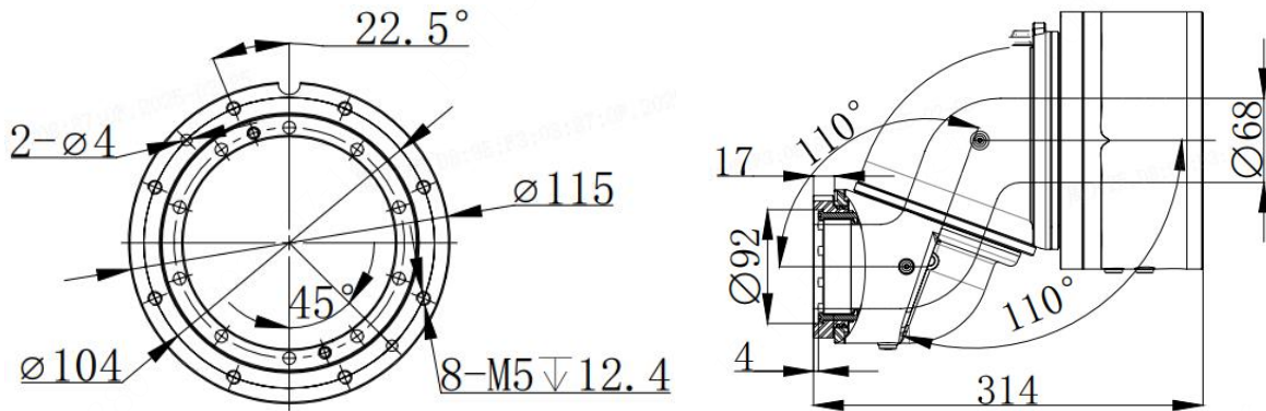
图 3-6 末端负载安装法兰尺寸
