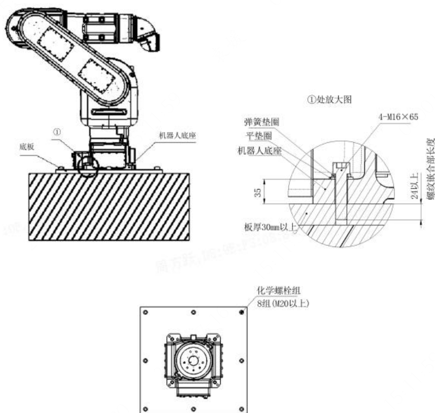
图 3-4 机器人安装举例
