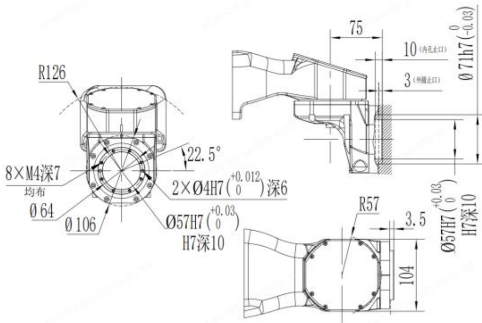
图 3-9 末端负载安装法兰尺寸
