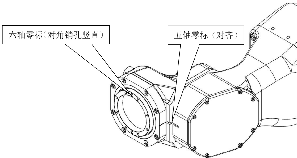
图 2-4 机械硬限位位置及零标位置
