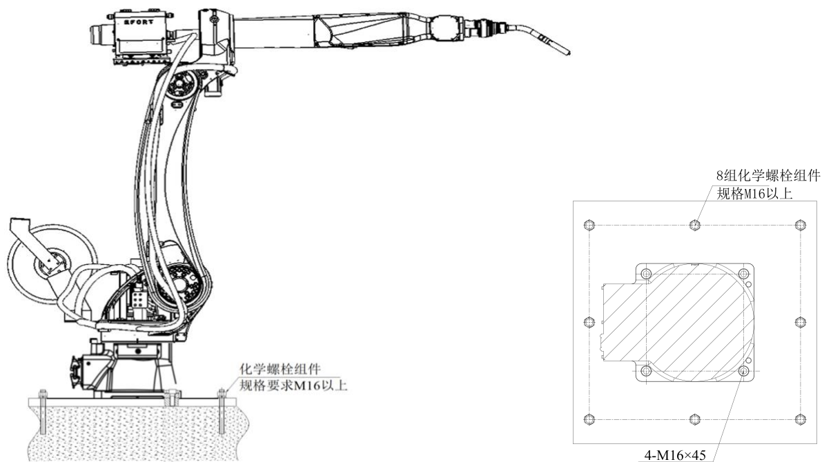
图 3-6 机器人安装举例
