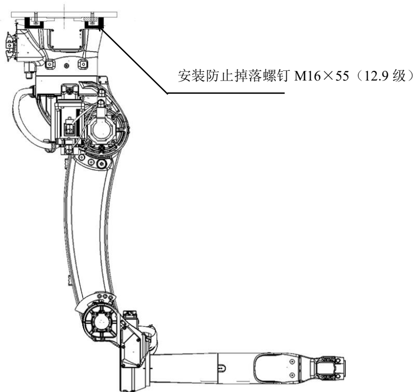
图 3-7 倒挂安装
