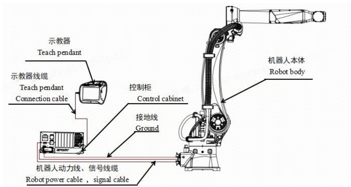
图 2-1 ARC12-2000 工业机器人系统构成
