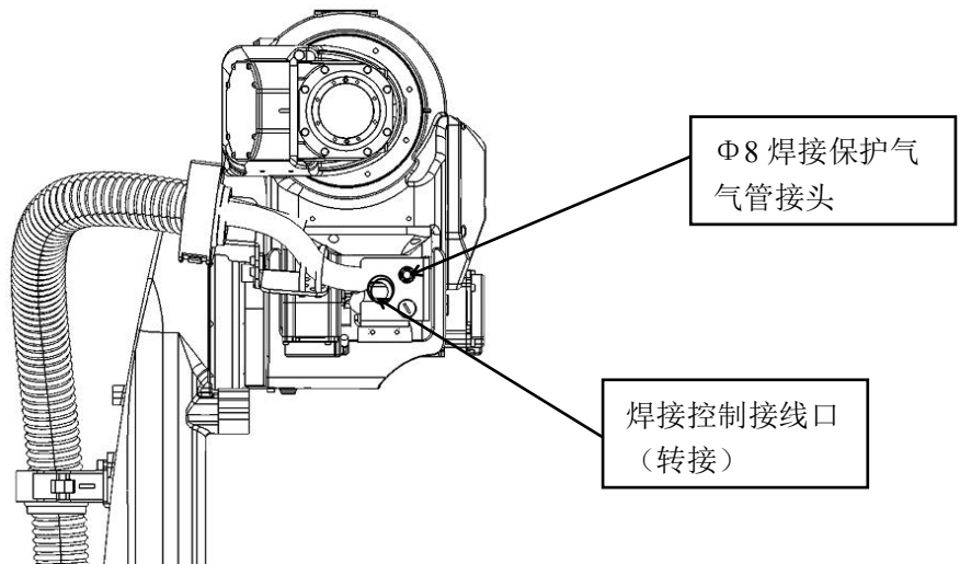
图 3-12 电机座部分气路及信号线接口
