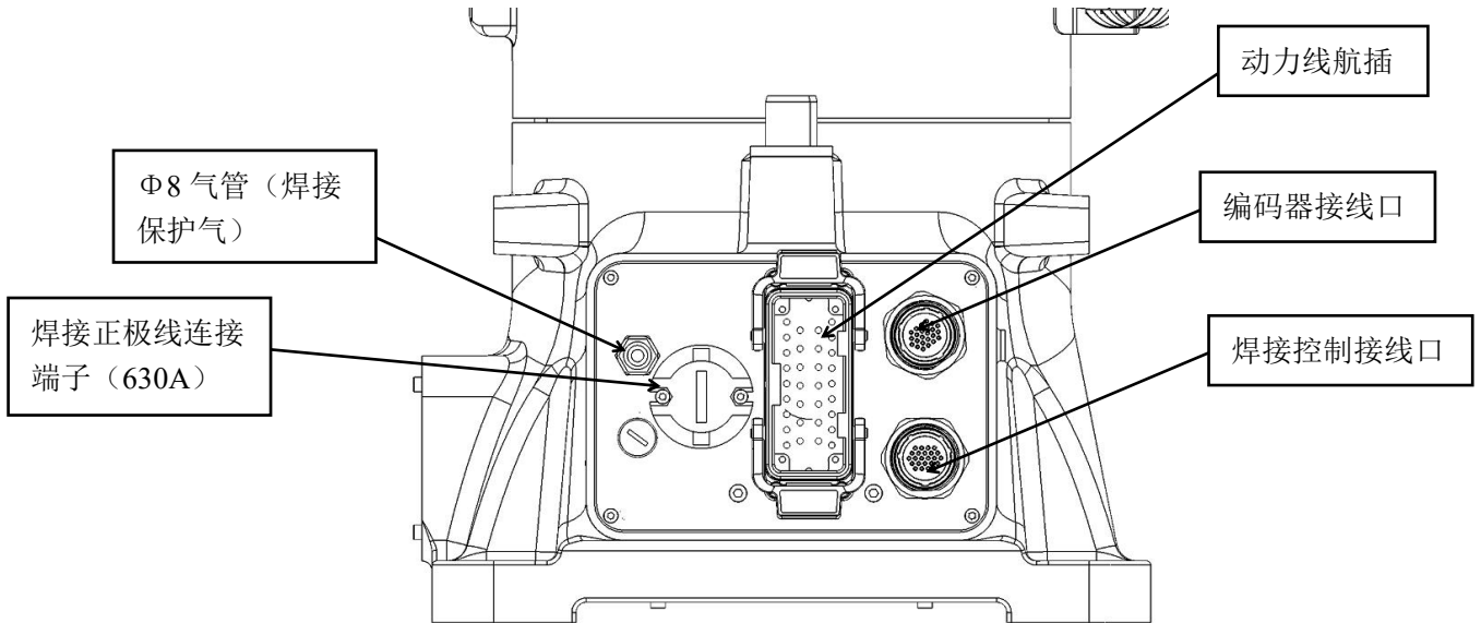
图 3-11 底座部分气路及信号线接口
