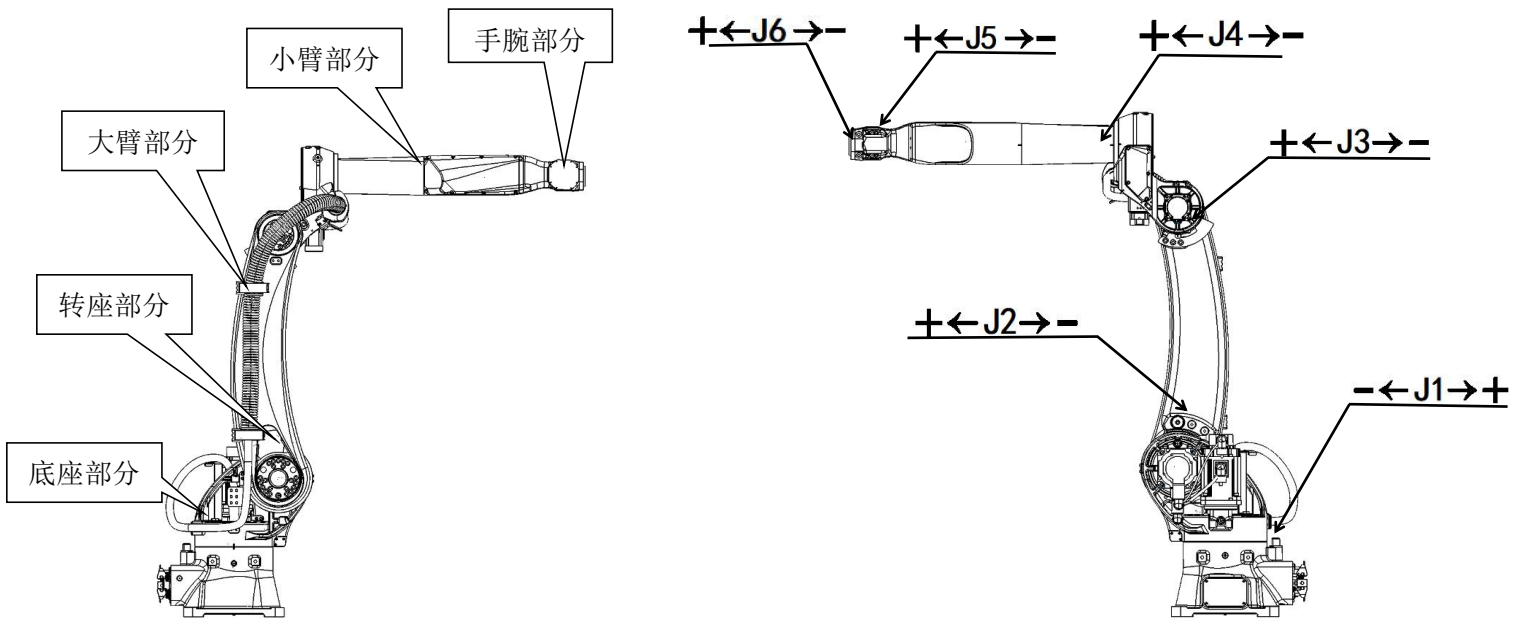
图 2-3 ARC12-2000 机械本体组成部分
