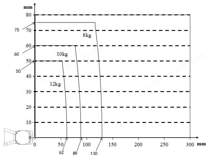
图 2-6 ARC12-2000 手腕轴转矩图
