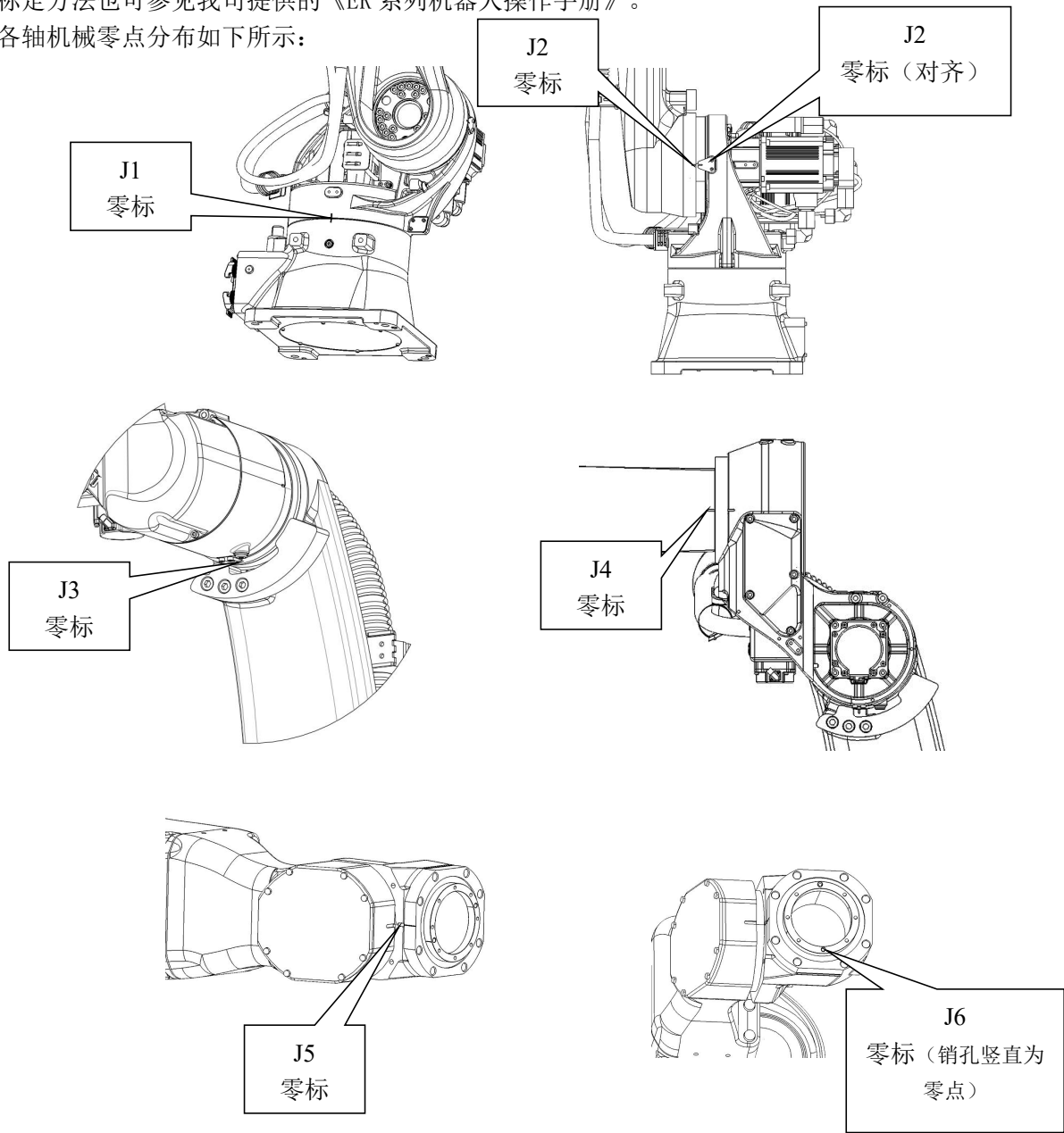
图 4-3 机器人零点位置图
