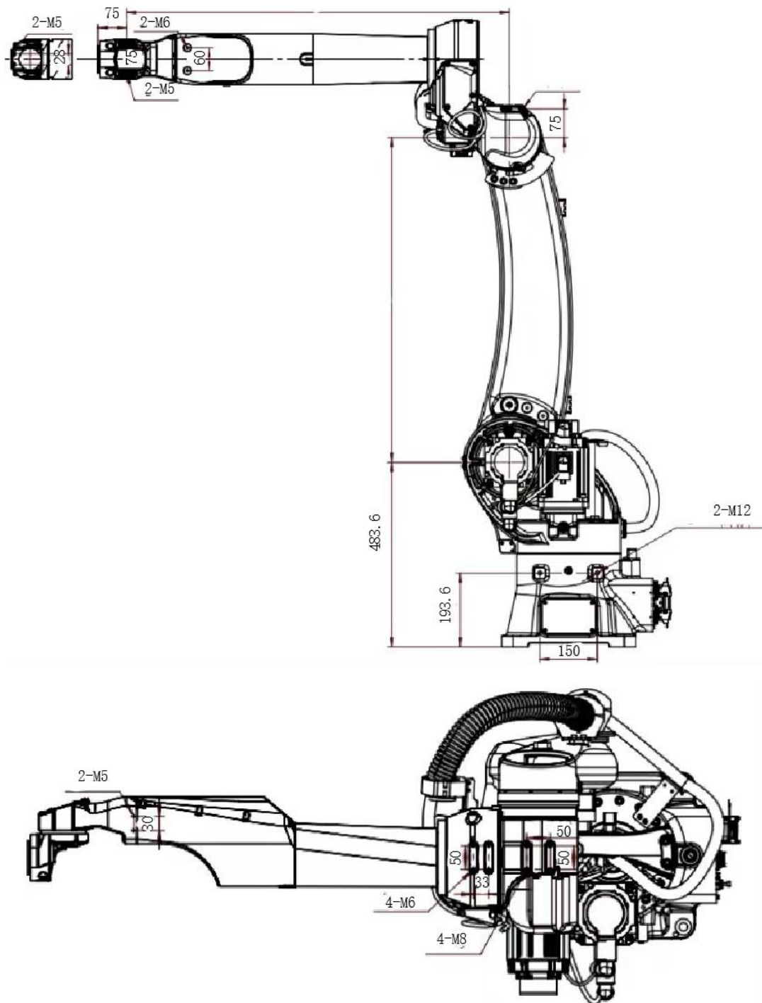
图 3-10 外围安装尺寸图
