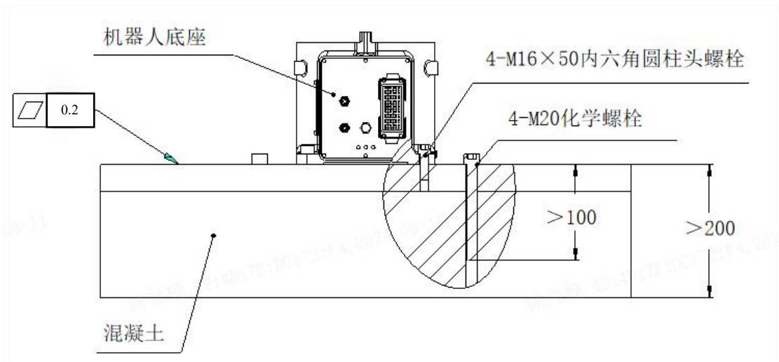
图 3-3 地面安装
