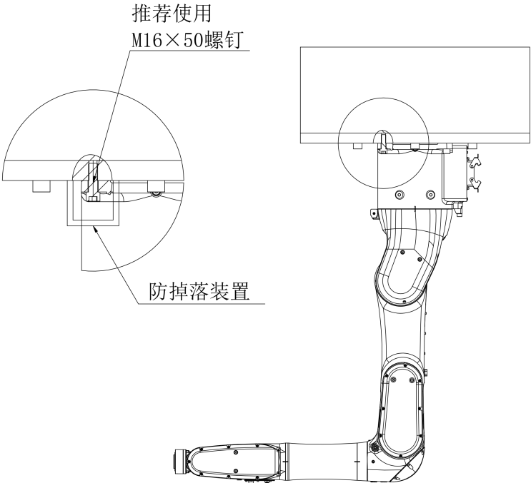
图 3-4 倒挂安装
