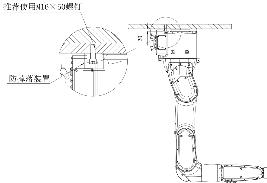
图 3-4 倒挂安装
