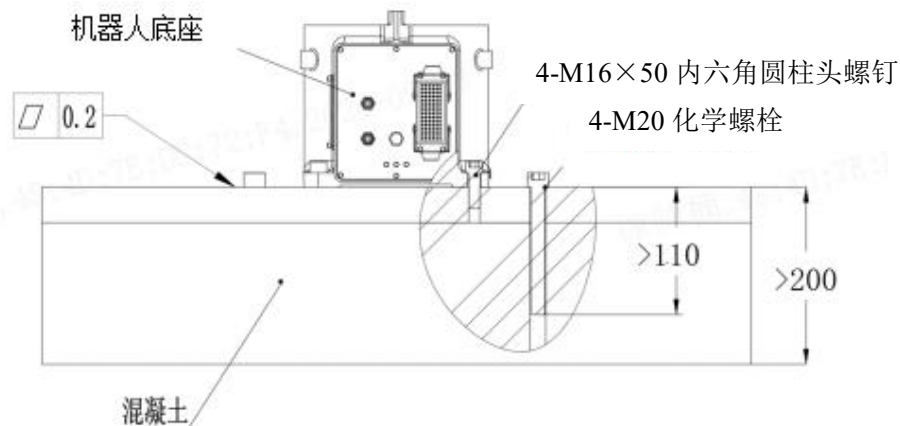
图 3-3 地面安装
