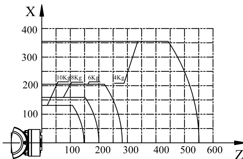
图 2-6 ER10-1100 手腕轴扭矩图
