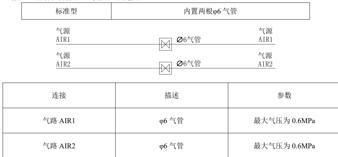
图 3-8 标准型气原理图
