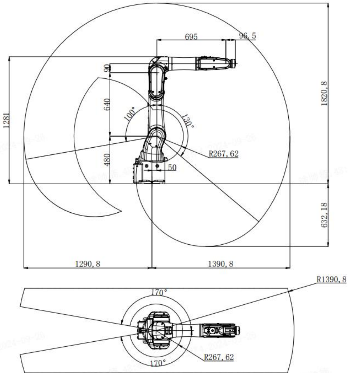
图 2-5 机器人工作空间图
