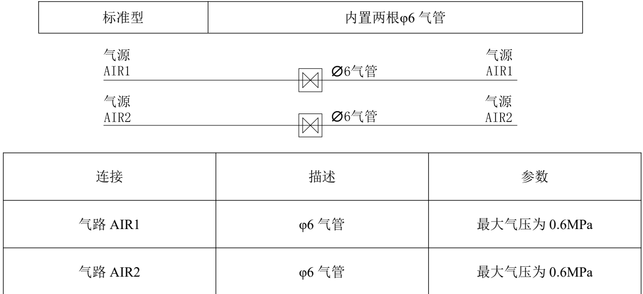
图 3-8 标准型气原理图
