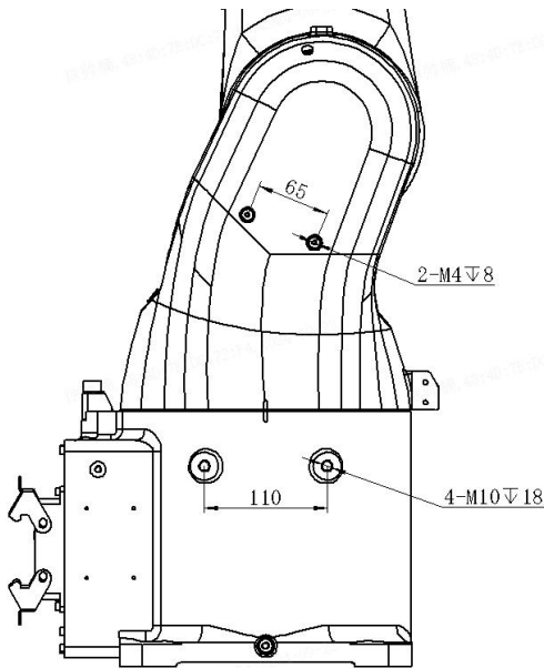
底座部分外部接口
