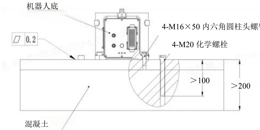
图 3-3 地面安装
