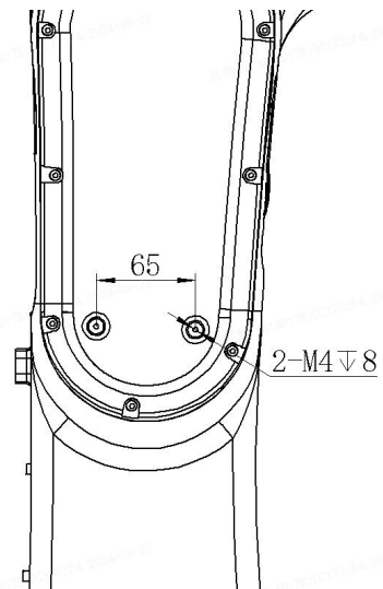
大臂部分外部接口
