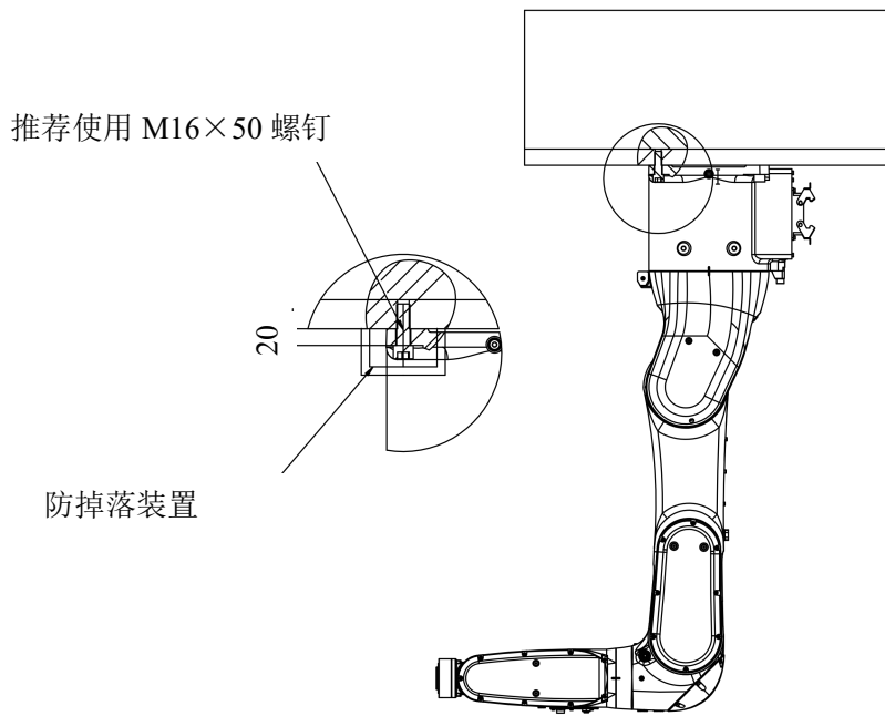
图 3-4 倒挂安装
