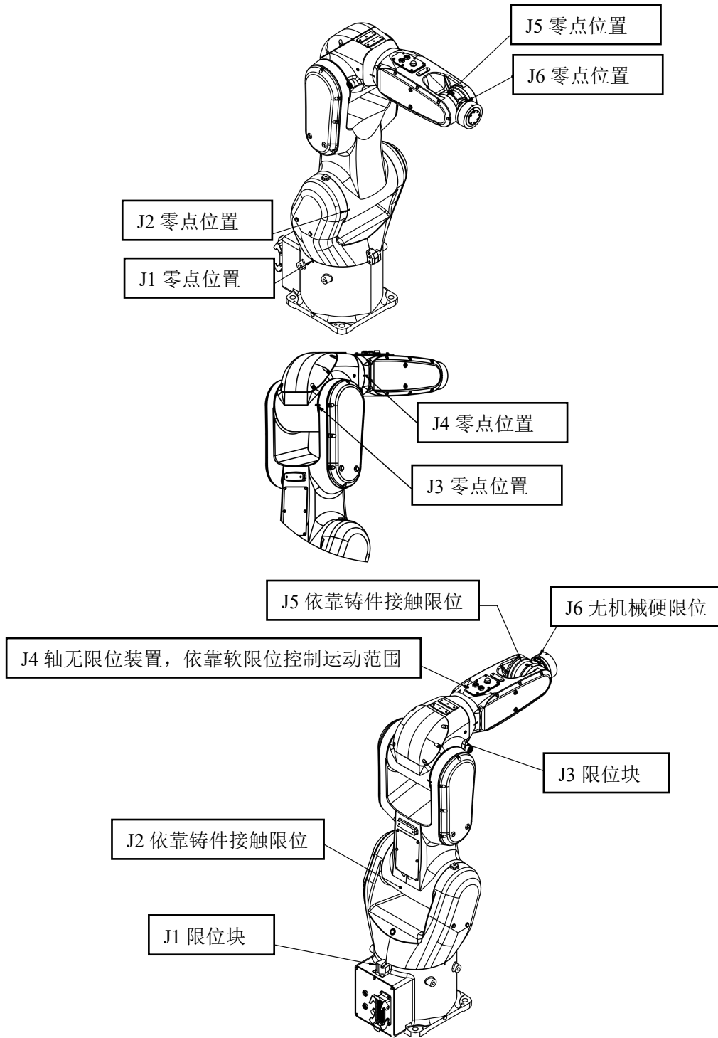
图 2-4 机械硬限位位置及零标位置
