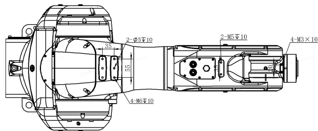
小臂部分外部接口
