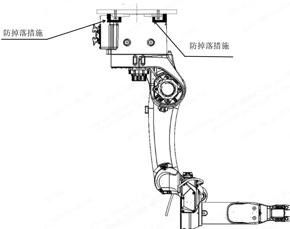
图 3-6 机器人倒装案例
