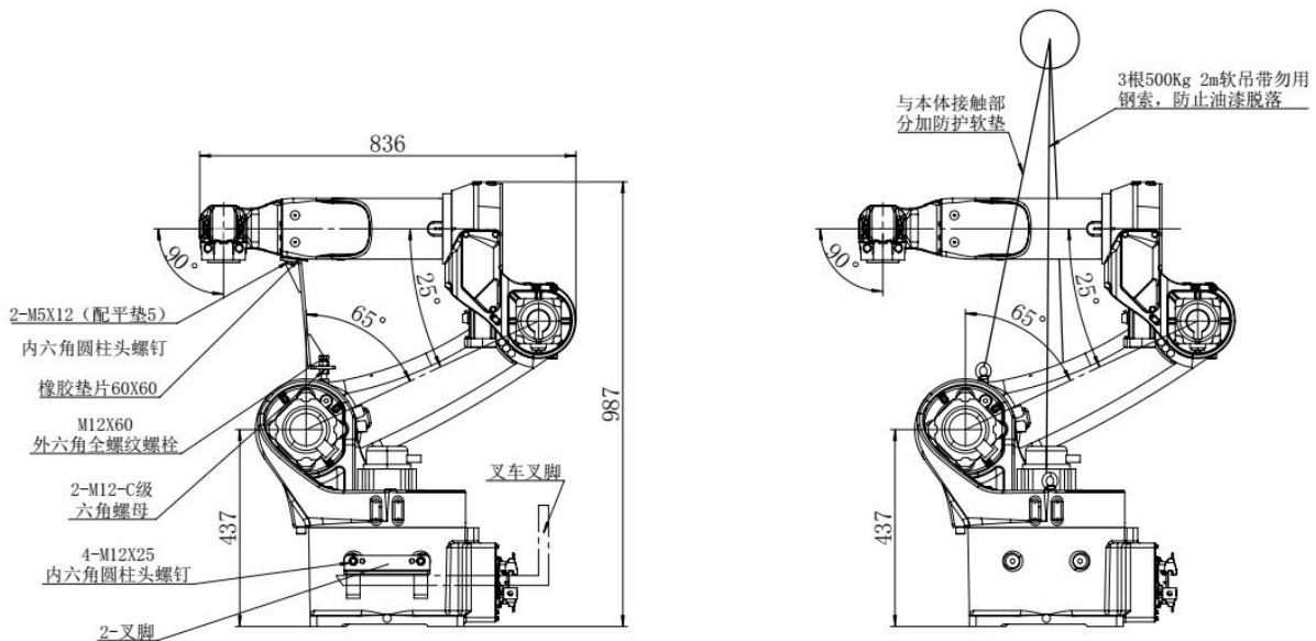
图 3-3 转运示意图（左侧叉车转运、右侧行车吊装）
