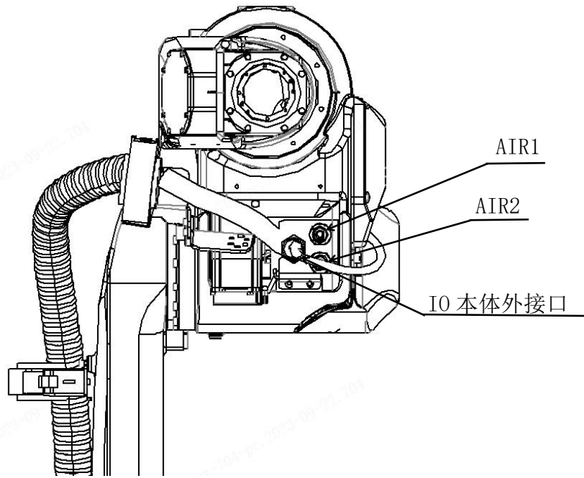
图 3-11 电机座部分气路及信号线接口
