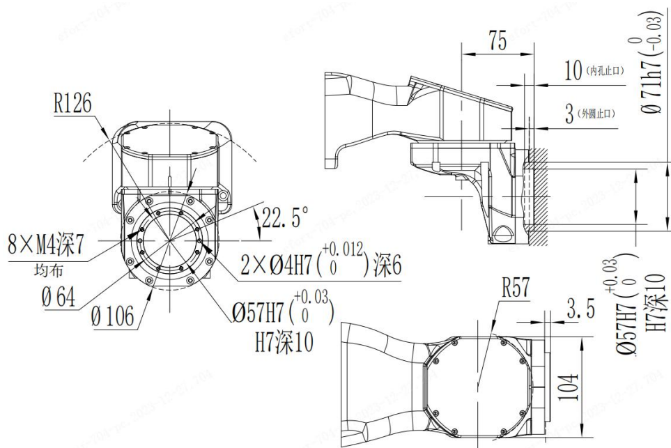
图 3-7 末端负载安装法兰尺寸
