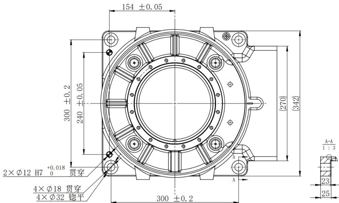
图 3-4 机器人底座尺寸
