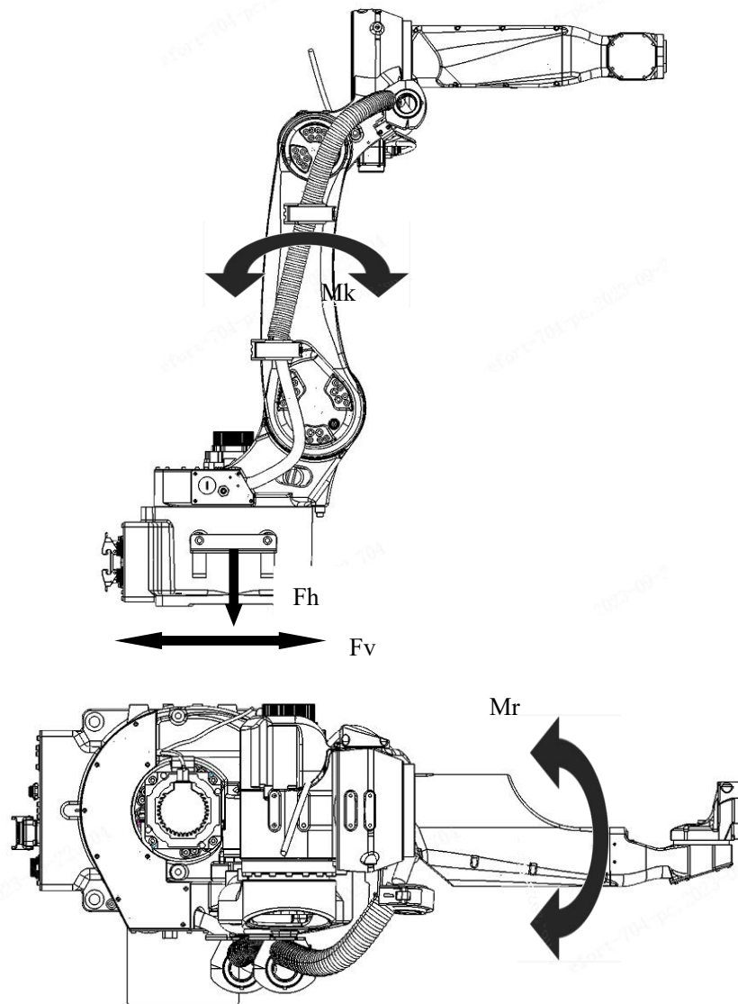
图 3-7 机器人受力图
