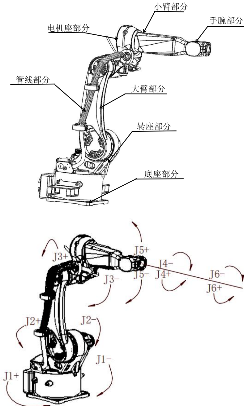
图 2-3 ER15H-1400 机械本体组成部分
