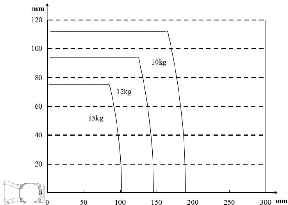
图 2-6 ER15H-1400 手腕转矩图
