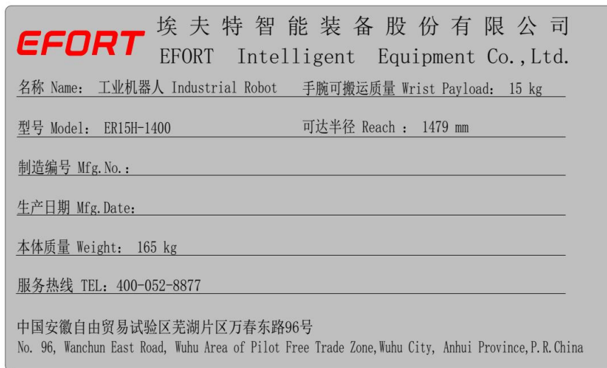
图 2-2 机器人本体铭牌
