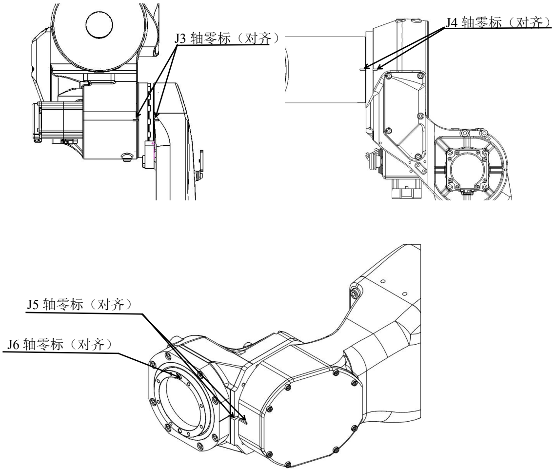
图 2-4 机械硬限位位置及零标位置
