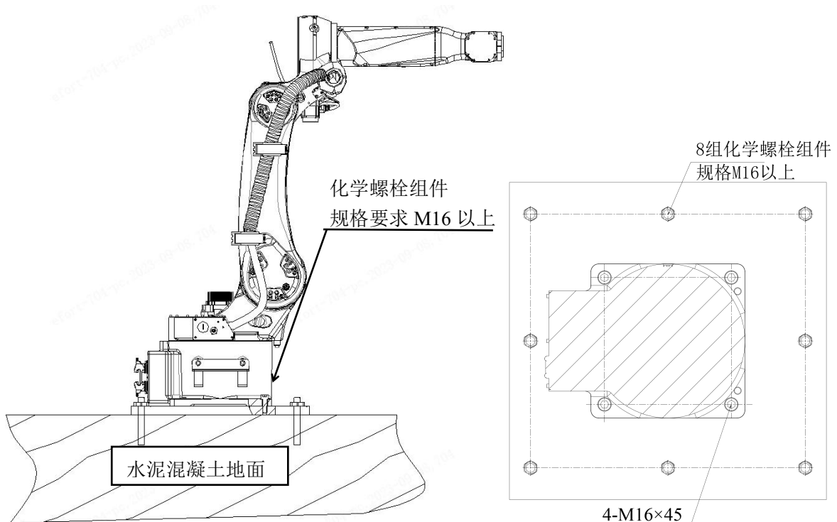
图 3-5 机器人安装举例
