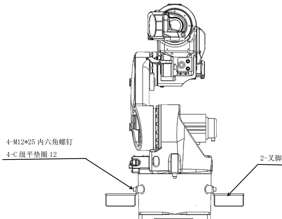
图 3-2 叉脚安装示意图
