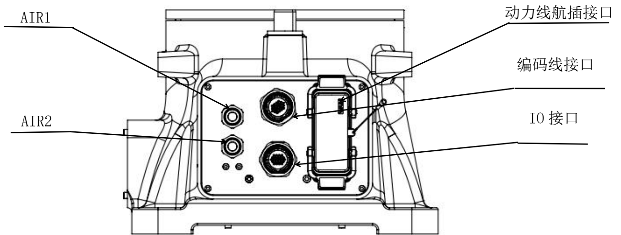
图 3-10 底座部分气路及信号线接口
