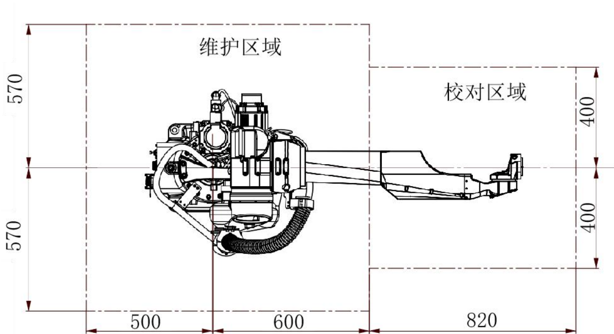
图 4-2 维护及使用区域
