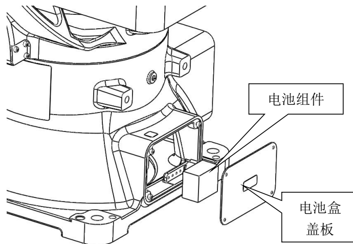
图 4-4 机器人电池组位置图
