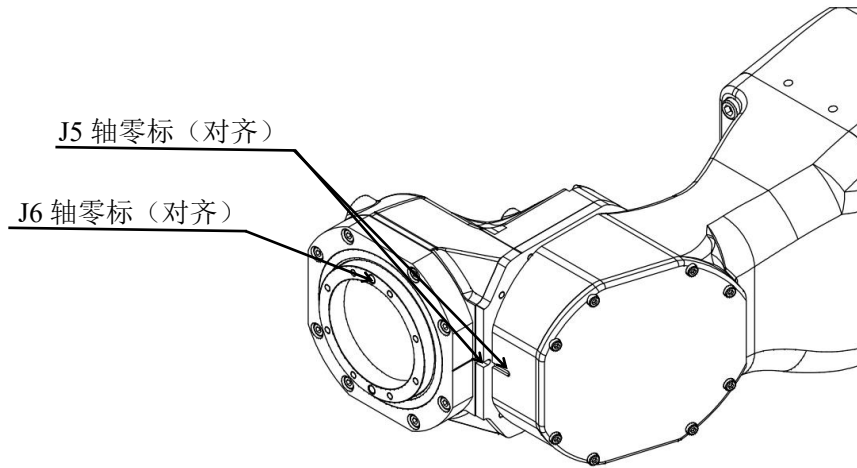
图 2-4 机械硬限位位置及零标位置
