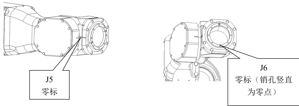
图 4-3 机器人零点位置图
