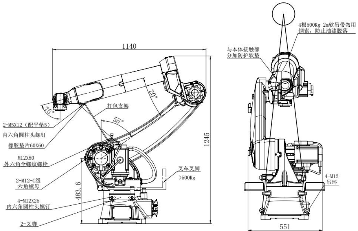
图 3-3 转运示意图（左侧叉车转运、右侧行车吊装）
