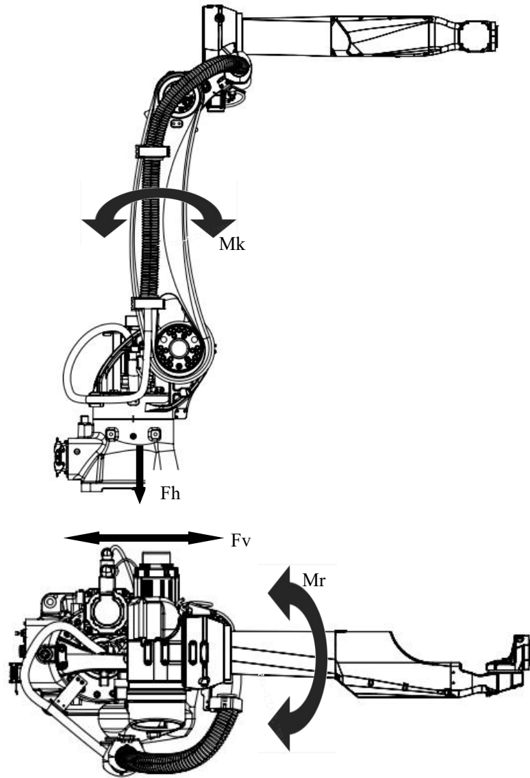
图 3-6 机器人受力图
