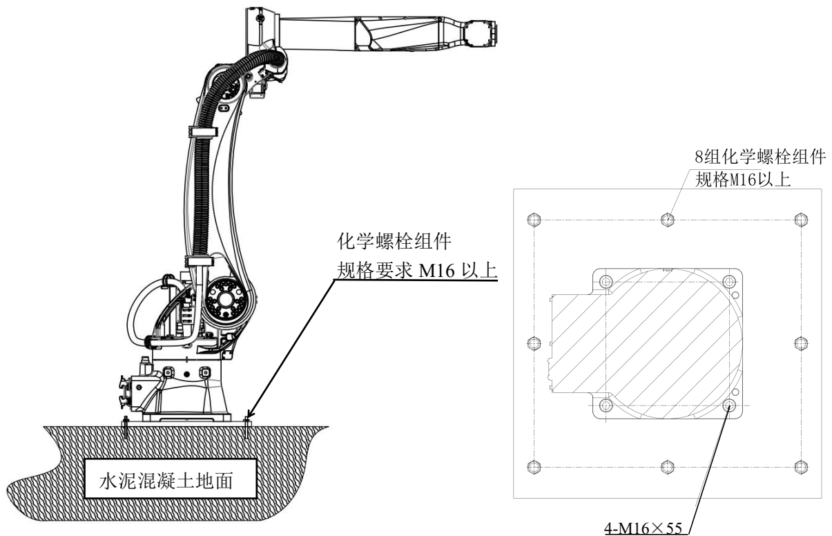
图 3-5 机器人安装举例
