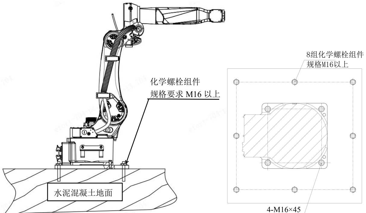
图 3-5 机器人安装举例
