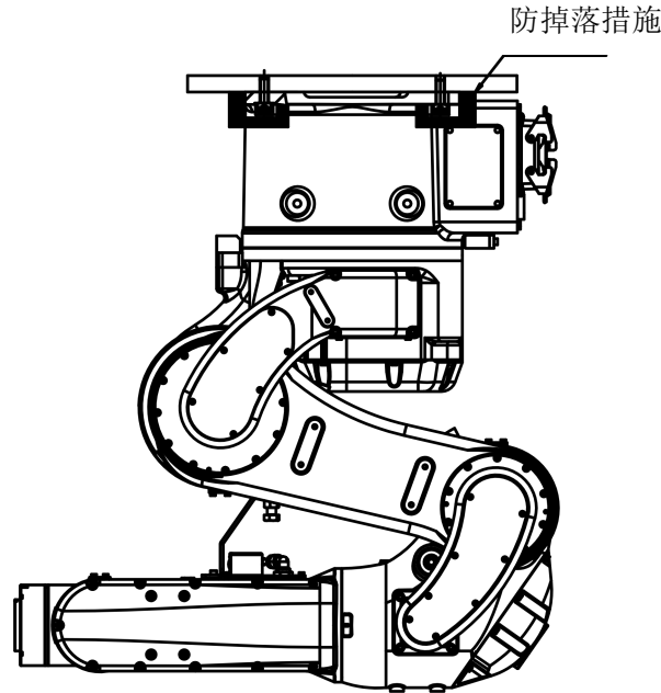
图 3-8 倒挂安装
