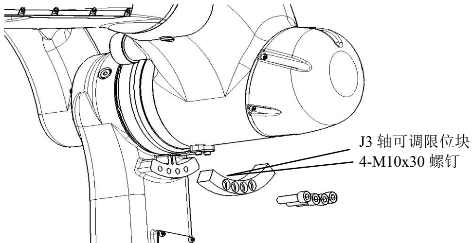
图 2-5 J3 轴可调限位图
