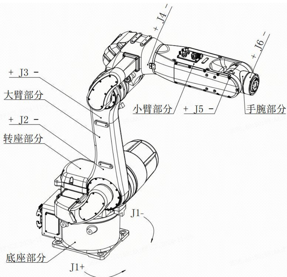
图 2-3 ER20-1100 机械本体组成部分
