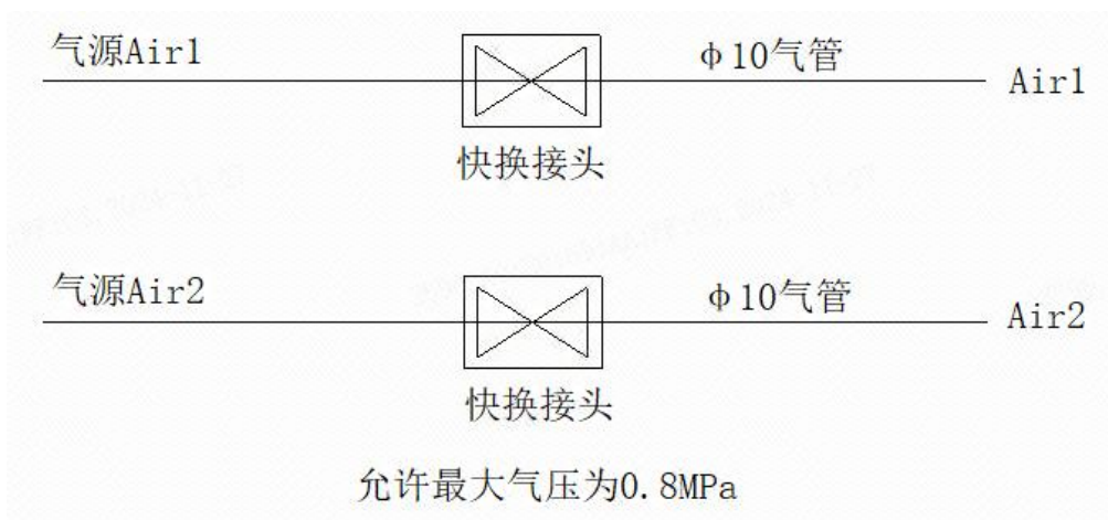
图 3-14 外接气管和信号线规格
