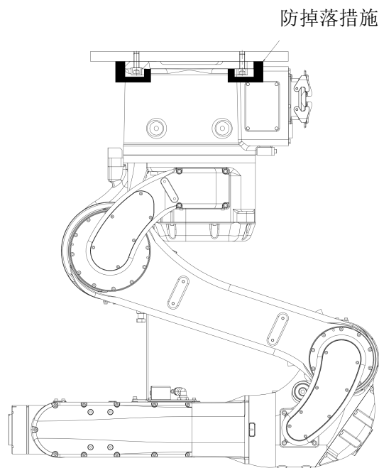
图 3-8 倒挂安装
