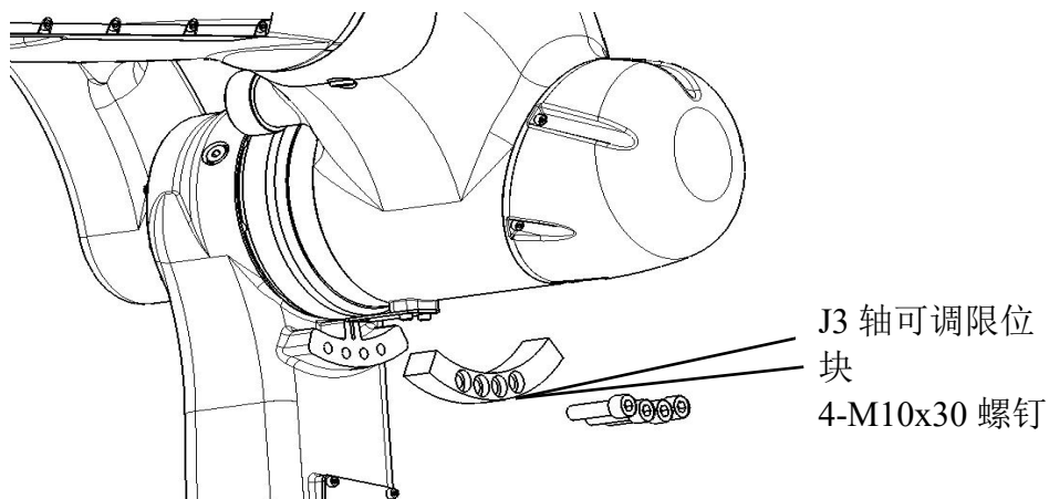
图 2-5 J3 轴可调限位图
