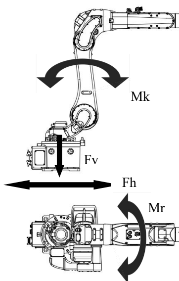
图 3-9 机器人受力图
