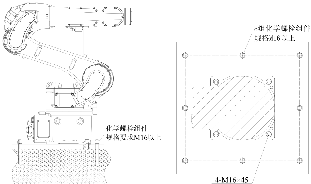
图 3-7 机器人安装举例
