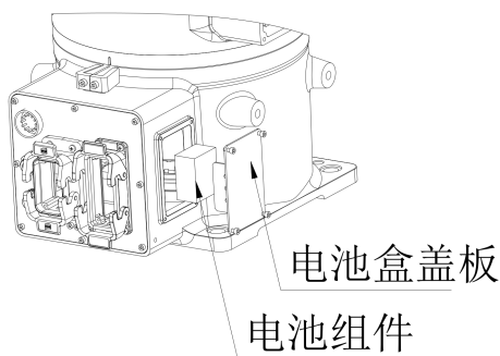
图 4-5 机器人电池组位置图
