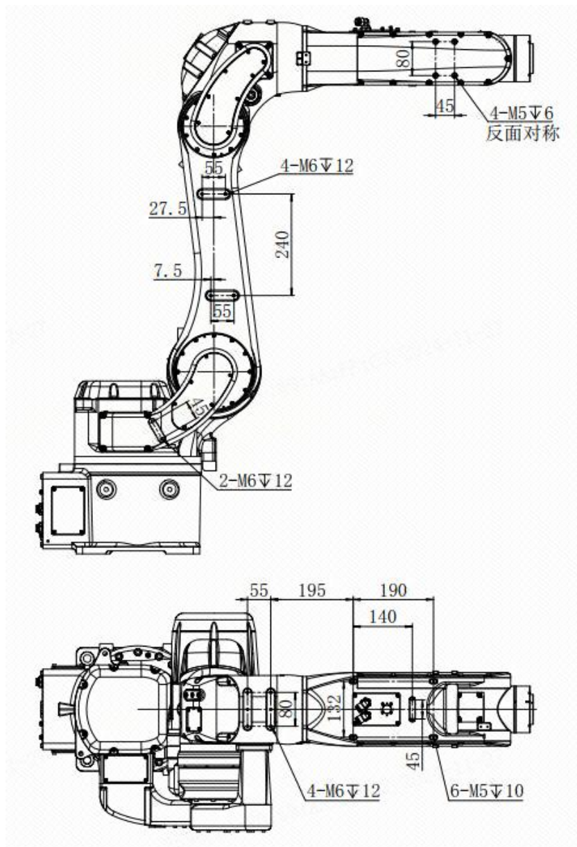
图 3-11 外围安装尺寸图
