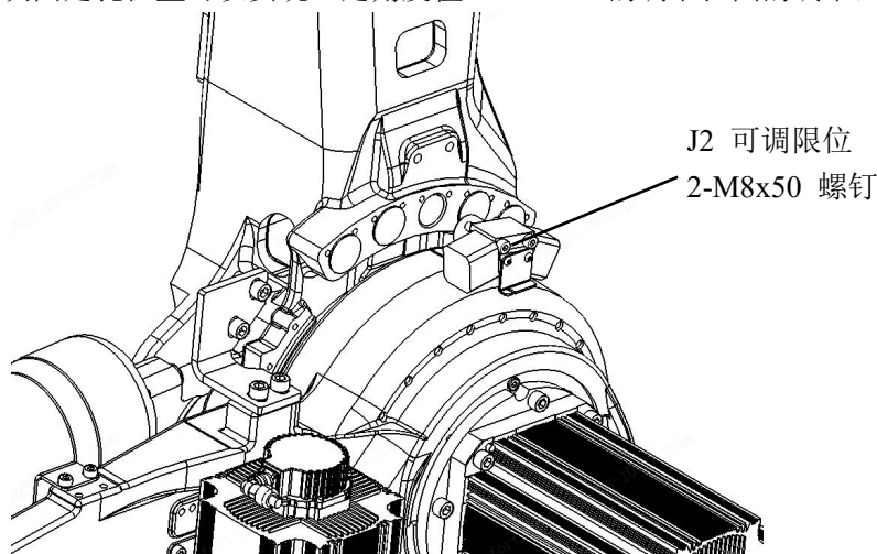
图 2-8 J2 轴可调限位图
