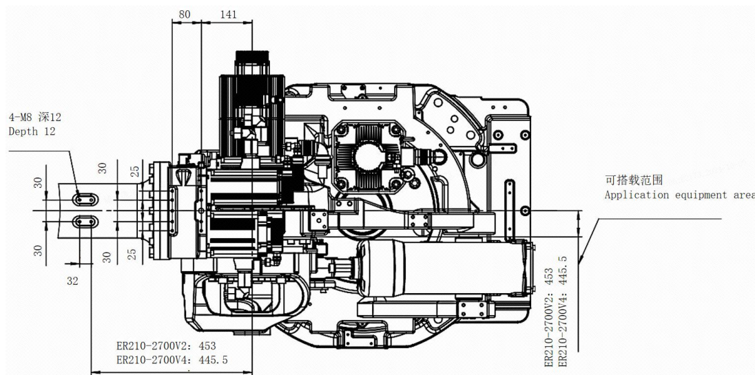
图 3-10 电机座/小臂杆上安装外部件尺寸图
