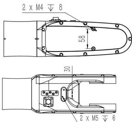
图 3-10 小臂杆上安装外部件尺寸图
