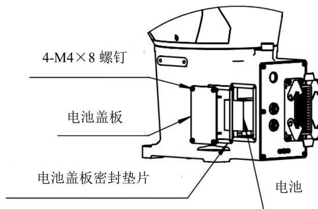
图 4-4 机器人电池组位置图
