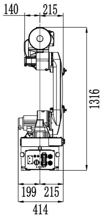
Base mounting size diagram 底座安装尺寸图
