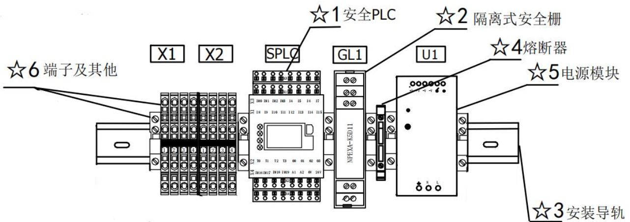
图 2-4 防爆电柜内部电气元器件布局
