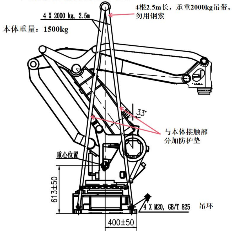
图 3-1 吊装搬运示意图
