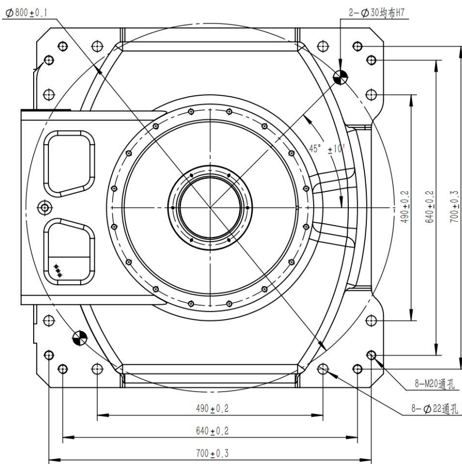
图 3-3 机器人底座尺寸
