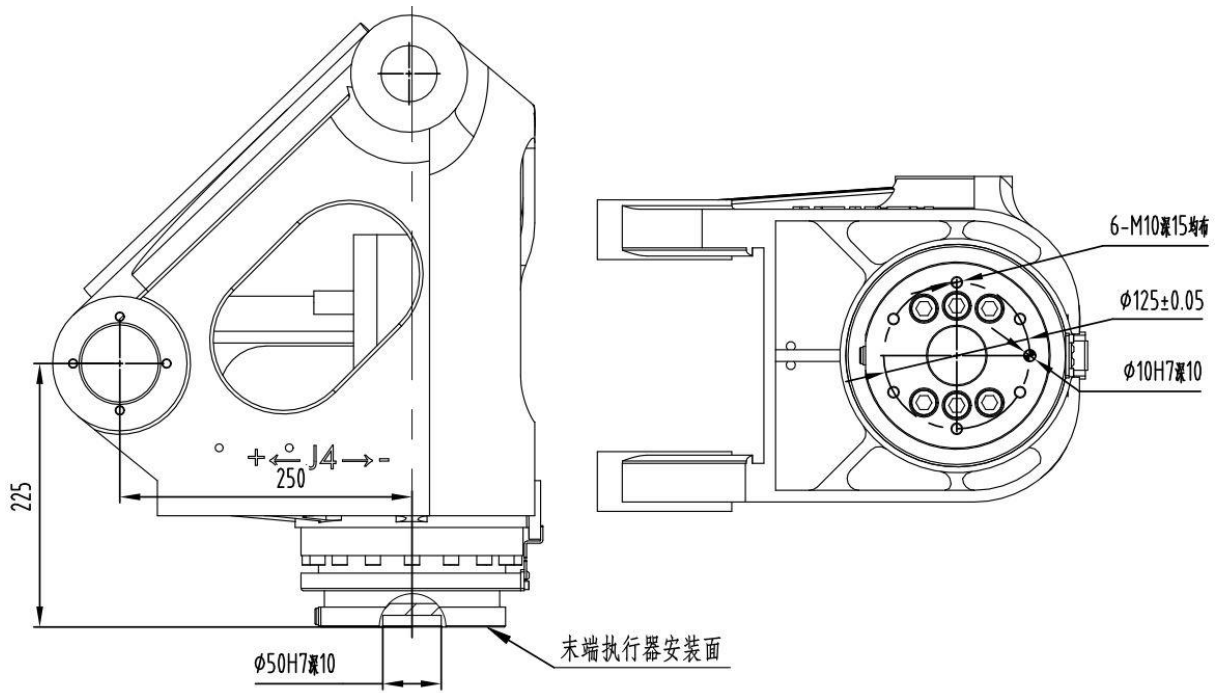
图 3-6 末端负载安装法兰尺寸
