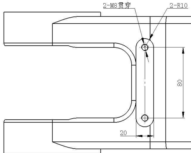
图 3-9 小臂杆上安装外部件尺寸图
