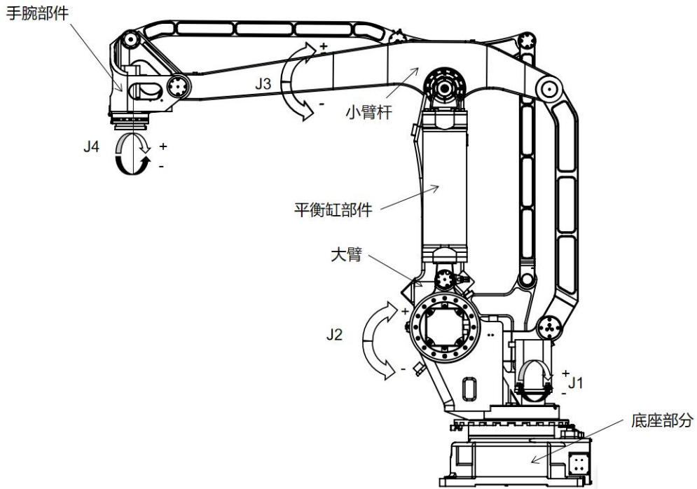
图 2-3 ER180-4-3200 机械本体组成部分
