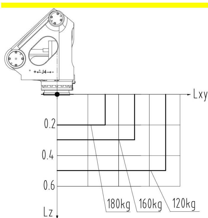
图 2-6 ER180-4-3200 手腕轴扭矩图
