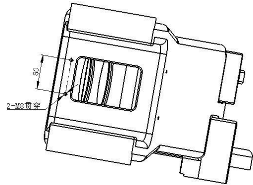
图 3-8 大臂上安装外部件尺寸图
