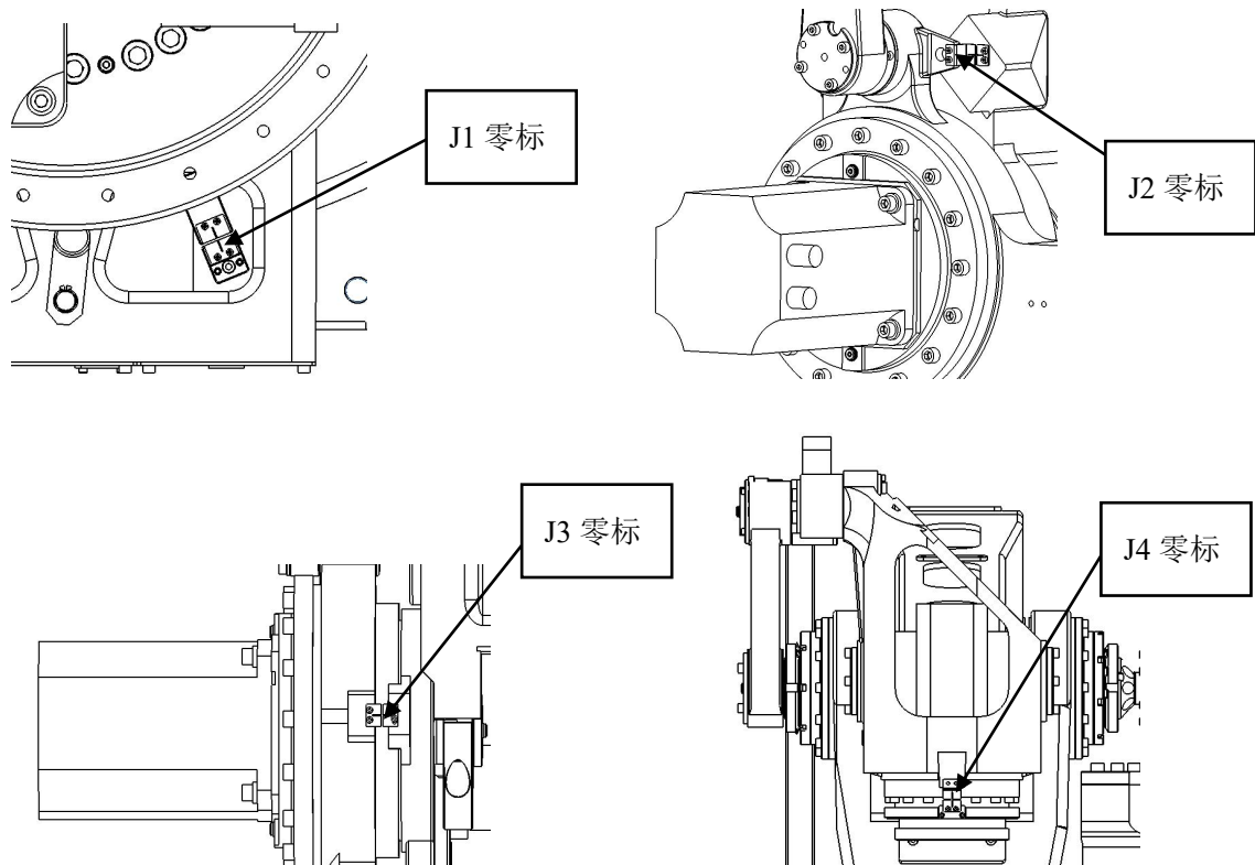
图 4-3 机器人零点位置图
