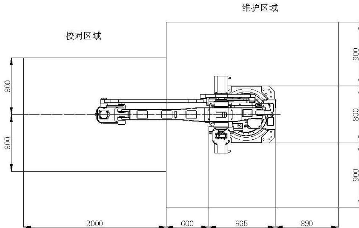
图 4-2 维护及使用区域
