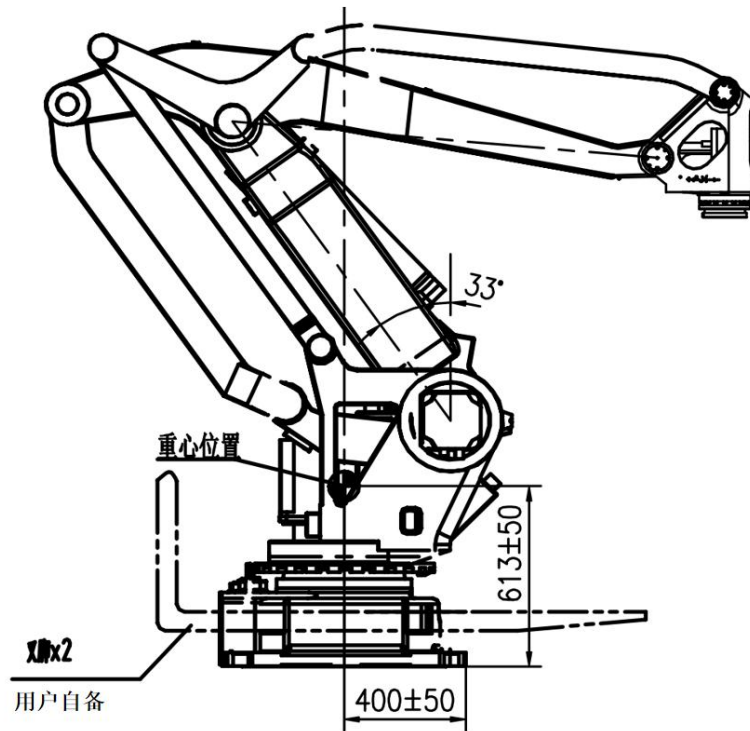
图 3-2 叉车搬运示意图
