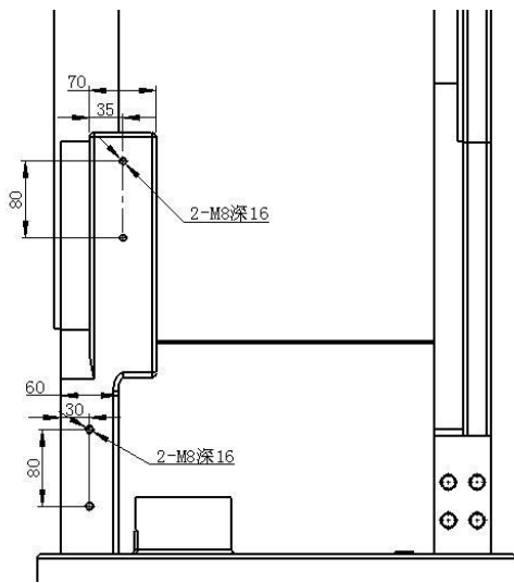
图 3-7 转座上安装外部件尺寸图
